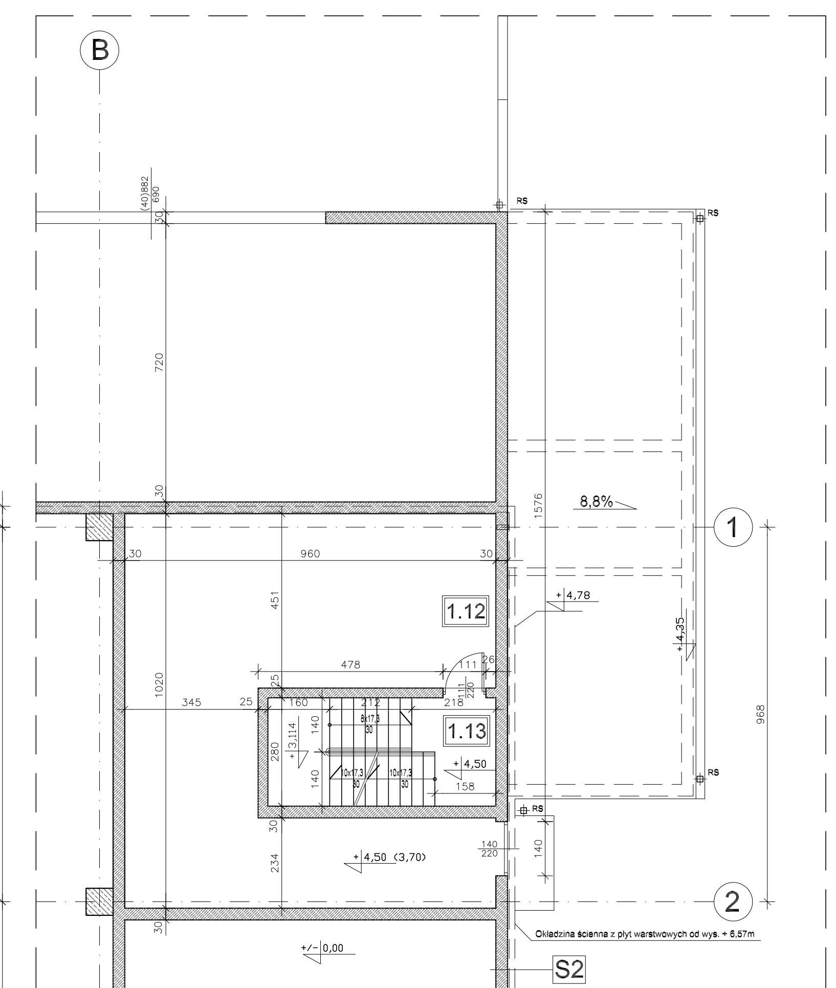
Zestawienie pom. 1 PIĘTRA (poziom + 4,50)
