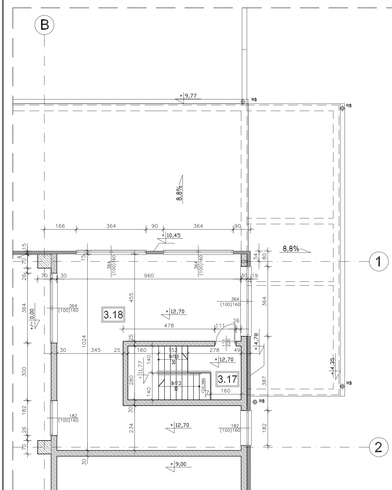
Zestawienie pom. 3 PIĘTRA (poziom + 12,70)
