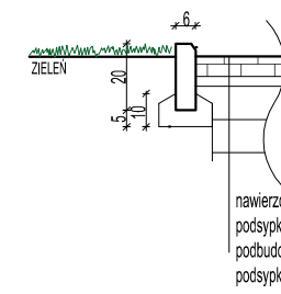
OBRZEŻE BETONOWE 6cm
