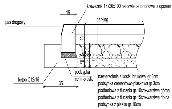
KRAWĘŻNIK BETONOWY WTOPIONY
