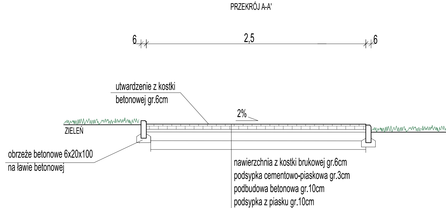
OBRZEŻE BETONOWE 6cm
