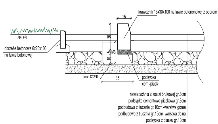
KRAWĘŻNIK BETONOWY WYSTĄJĄCY
