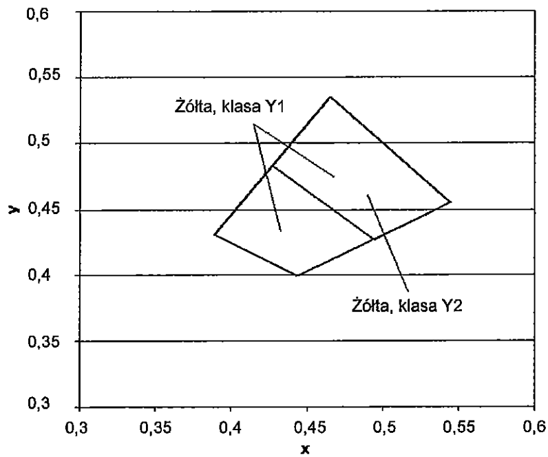
Rys.2. Współrzędne chromaticzności x, y dla barwy żółtej oznakowania
