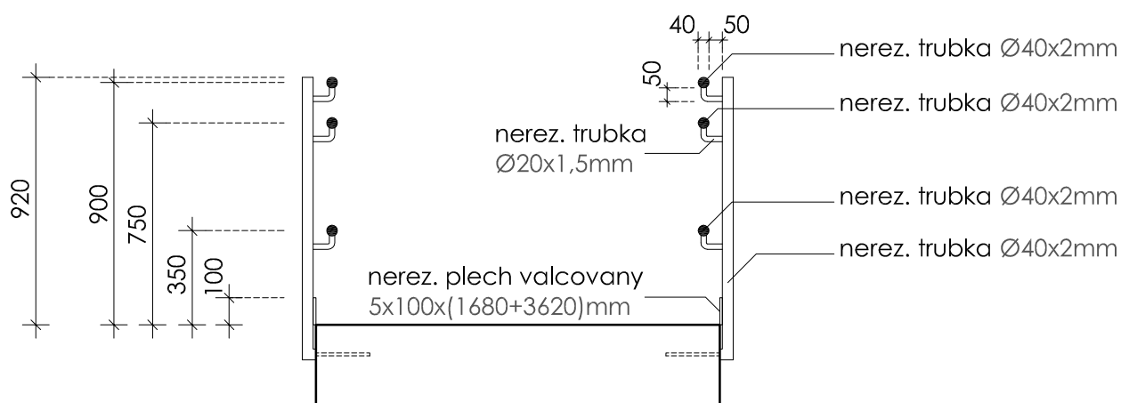
Zábradlie rampy - prierez profilov
