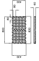
DETAIL ROŠTU
