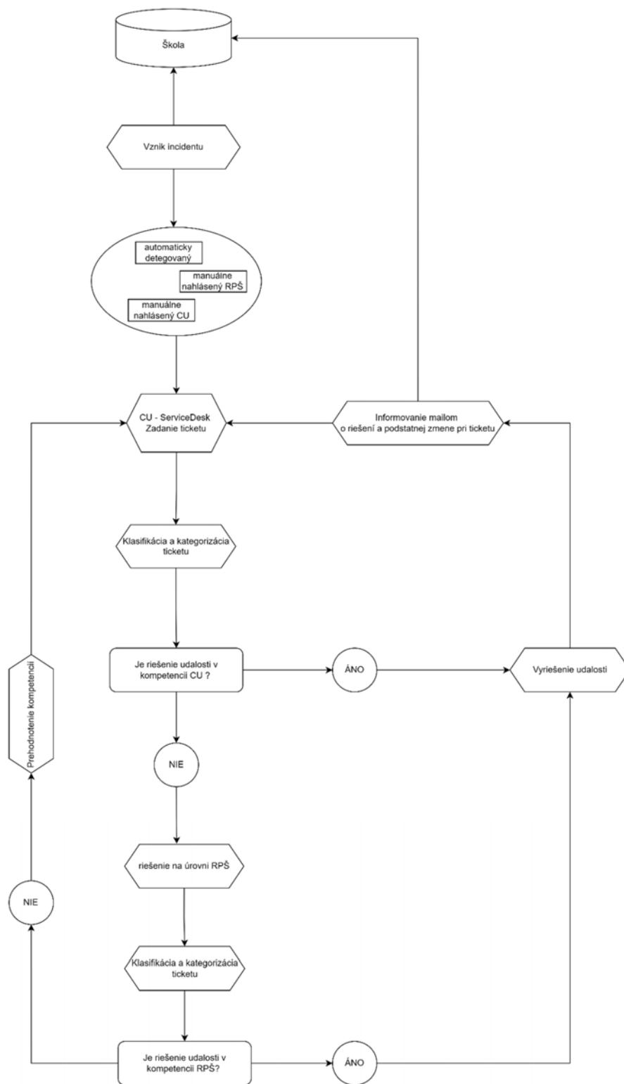
Obrázok 3: Proces spracovania incidentu
