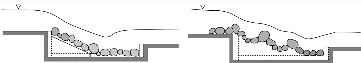
Rys. 97. Przebudowa stopni betonowych – bystrze z kamieni ułożonych na płycie dennej starego progu [Żelazo i Popek 2014]
