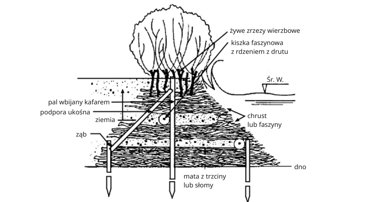
Rys. 57. Żywa tama faszynowa [Begemann i Schiechl 1999]
