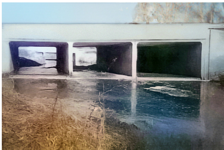
Fot. 124. Błędnie zaprojektowana rzędna dna ograniczająca migrację ryb podczas niżówek [Kosicki 2011]
