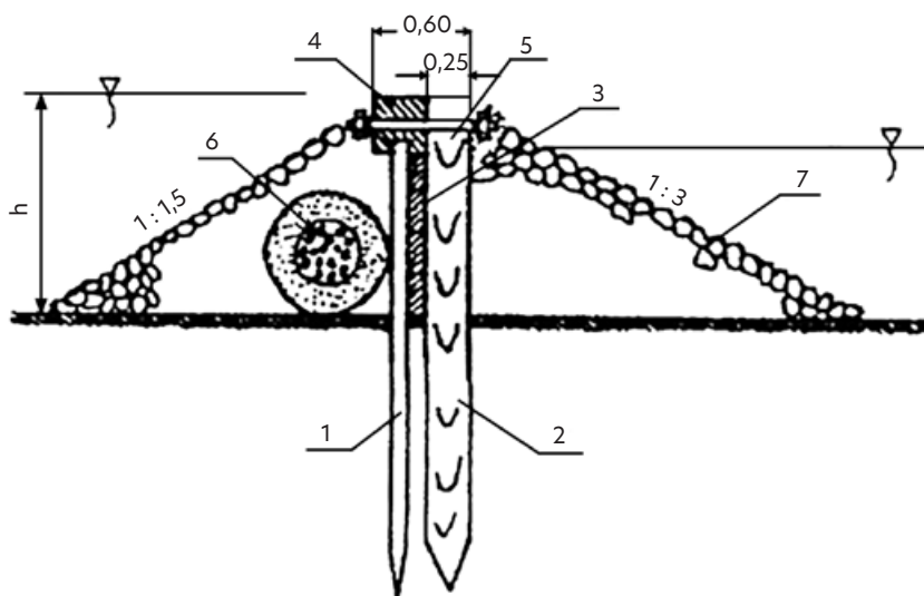
Rys. 44. Próg z walców faszynowych i narzutu kamiennego [Wołoszyn 1974]
