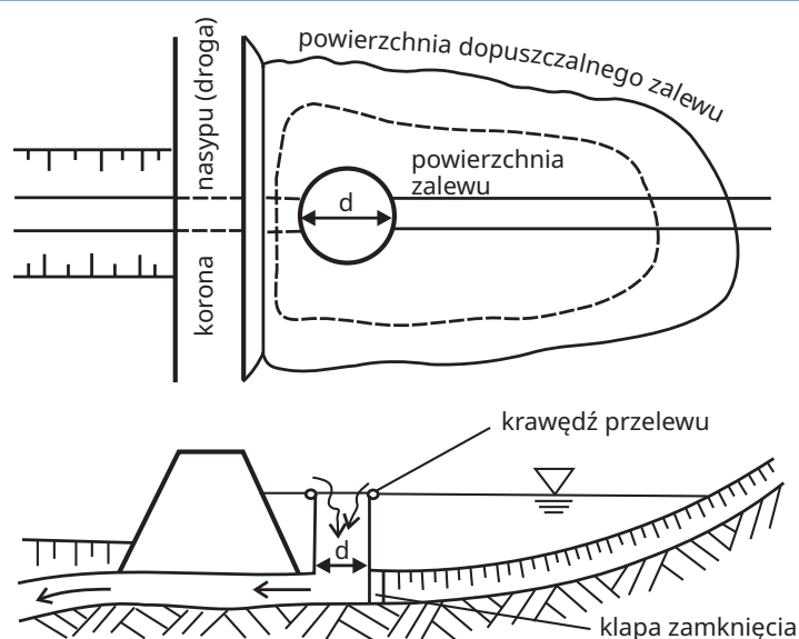
Rys. 51. Opóźniacz odpływu, rzut z góry i przekrój podłużny [opracowano na podstawie: Paluch i in. 2005]
