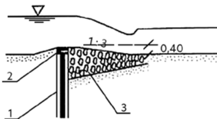
Rys. 36. Próg ze ścianki szczelnej [Dębski 1971]
