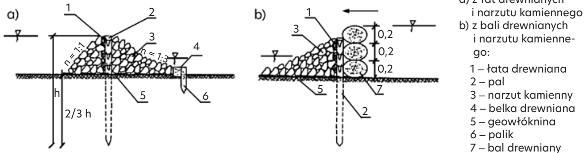
Rys. 42. Progi o konstrukcji mieszanej [Jędryka 2006]
