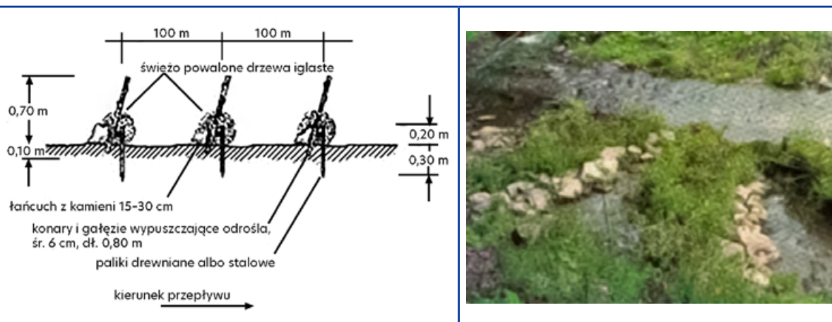
Rys. 59. i Fot. 61. Schemat żywych ostróg pośrednich [Begemann i Schiechtl 1999]
