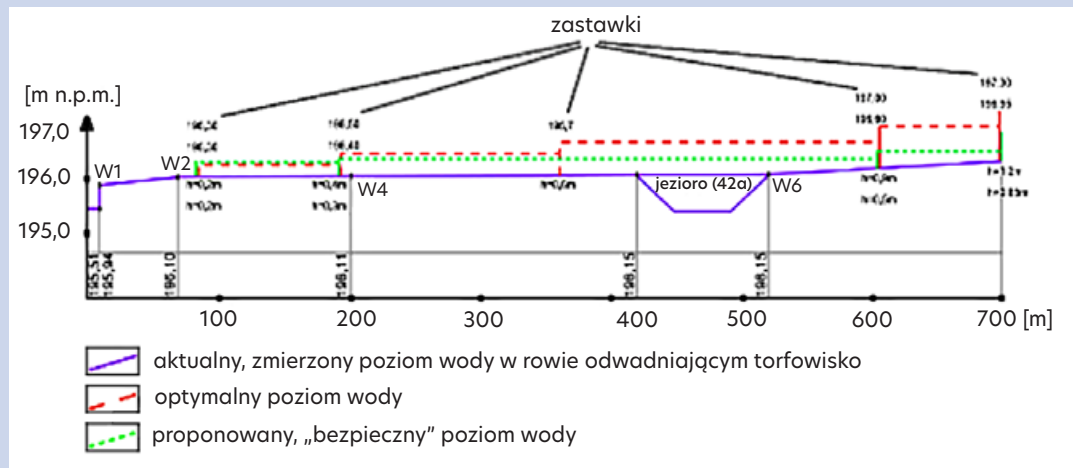
Rys. 23. Stopniowe podpiętrzanie wody na mokradle w ramach renaturyzacji prowadzonej przez Klub Przyrodników w rezerwacie „Jeziorka Chrościckie” (rys. P. Włodarczyk, na podstawie: Herbichowa i in. [2007])
