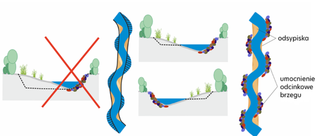
Rys. 6. Zachowanie morfologii koryta w pracach związanych z utrzymaniem wód (autor: Sz. Radosz, CKPŚ)
