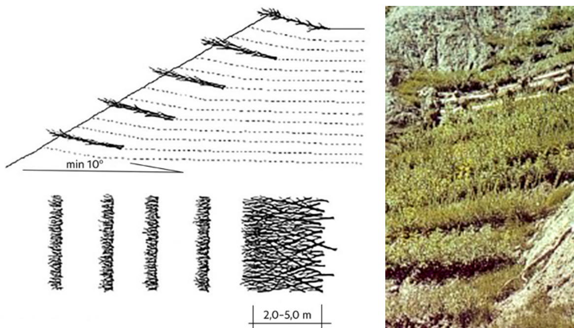
Rys. 66. i Fot. 64. Krzewiaste umocnienia tarasowe na skarpie/osuwisku [Begemann i Schiechtel 1999]
