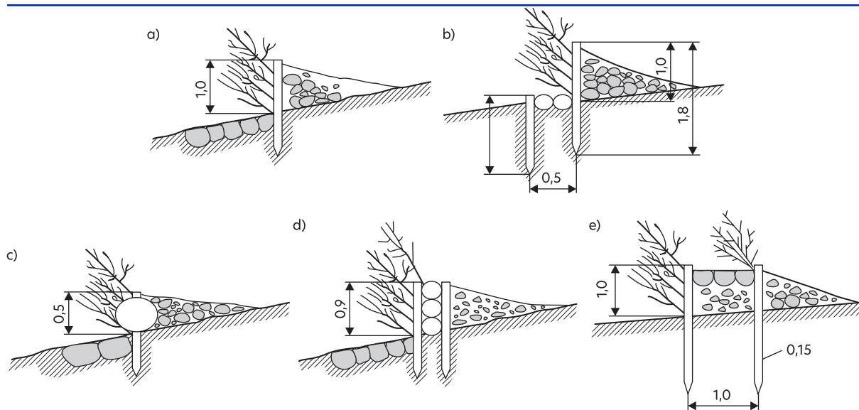
Rys. 99. Płotki drewniano-ziemne z nasadzeniami: a, b, c, d – pojedyncze, e – podwójne [opracowano na podstawie: Prochal 1968]
