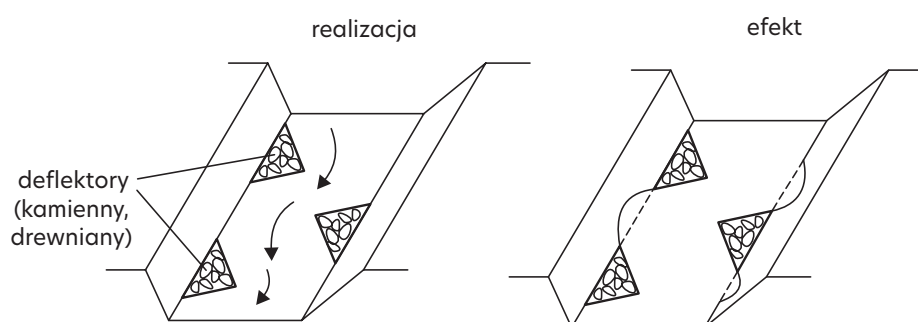
Rys. 53. Schemat naprzemiennego rozmieszczenia deflektorów/ostróg z materiałów naturalnych (rys. L. Książek)
