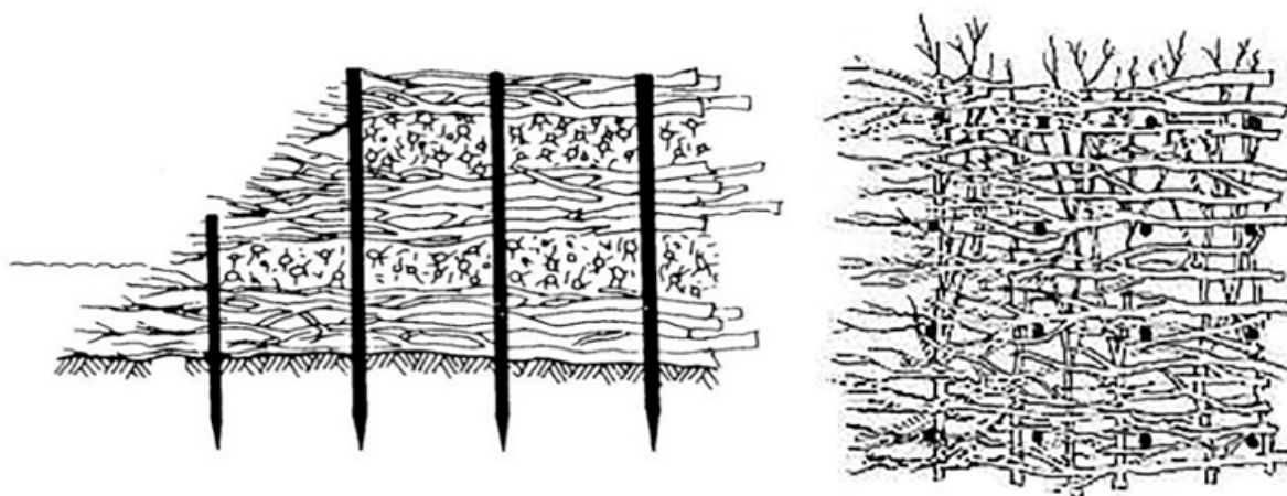
Rys. 76. Brzegoston krzyżowy z lewej – przekrój poprzeczny, z prawej – rzut z góry [Begemann i Schiechtl 1999]
