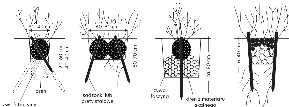
Rys. 63. Różne rodzaje drenów faszynowych [opracowano na podstawie: Begemann i Schiechtel 1999]
