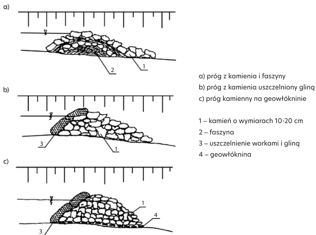
Rys. 40. Przykłady progów z kamienia [Mioduszewski 2003]
