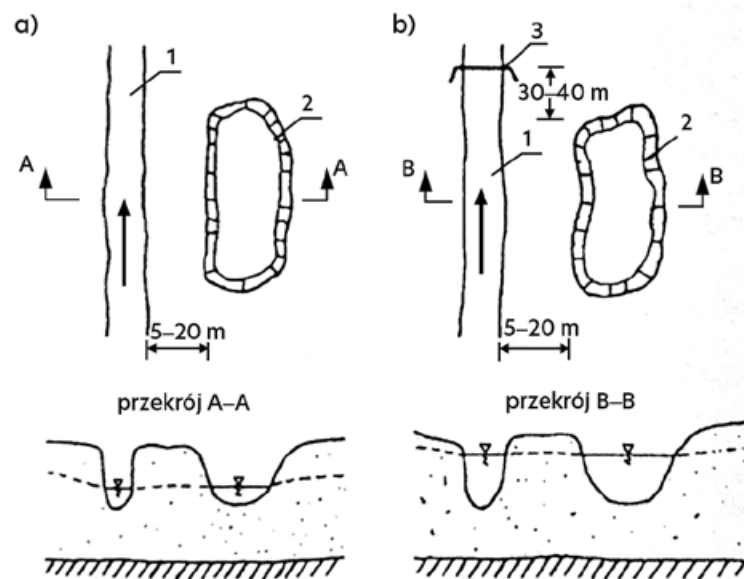
Rys. 13. Zbiornik zasilany infiltracyjnie z cieków: a) przy ciekach naturalnych, b) przy ciekach spiętrzonych [Mioduszewski 2014]
