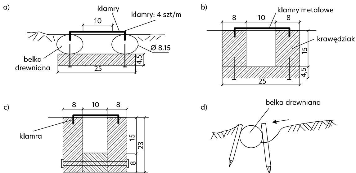
Rys. 101. Przekroje typowych wodospustów: a – drewniany z bali, b – drewniany z krawężniaków typ I, c – drewniany z krawężniaków typ II, d – z kamienia lub drewna [opracowano na podstawie: Drogi leśne 2006].
