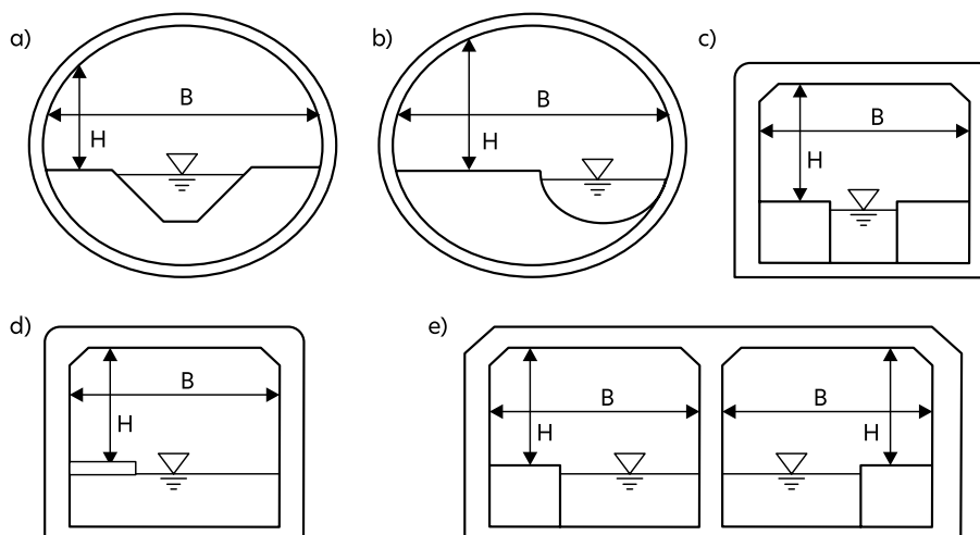
Rys. 90. Przepusty/przejścia zespolone: a) ze ścieżką dwustronną w przepusie kołowym, b) ze ścieżką jednostronną, c) ze ścieżką dwustronną w przepusie prostokątnym, d) ze ścieżką (półką) jednostronną w przepusie prostokątnym, e) ścieżki w przewodzie podwójnym [opracowano na podstawie: Bajkowski i Marzysz 2004]
