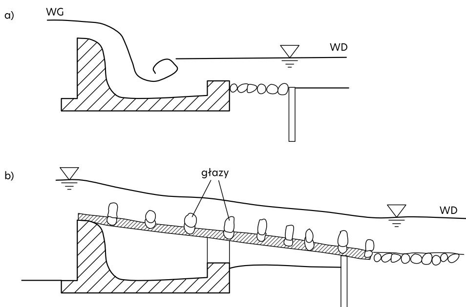
Rys. 96. Projekt przebudowy jazu stałego na przepławkę dla ryb [opracowano na podstawie: Mokwa i Wiśniewski 2008]
