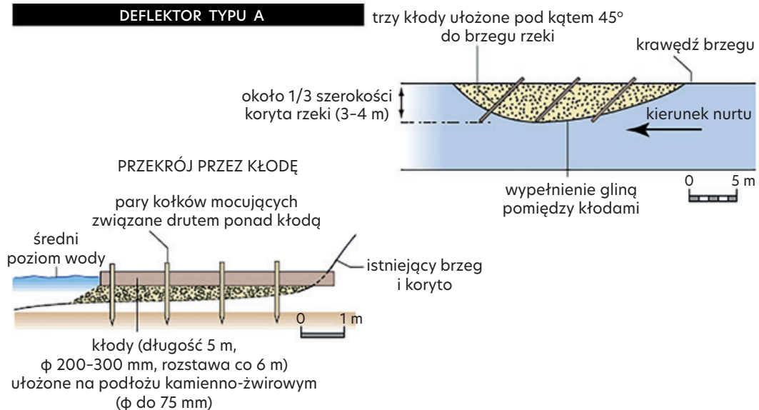
Rys. 54. Ostrogi z kłód drewna na podłożu kamiennie-żwirowym na przykładzie realizacji na rzece Skerne, Darlington, Anglia [Krukowski 2006]
