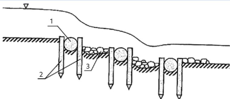
Rys. 45. Kaskada niskich progów drewnianych lub drewniano-faszynowych stabilizujących profil podłużny dna [Żelazo i Popka 2014]
