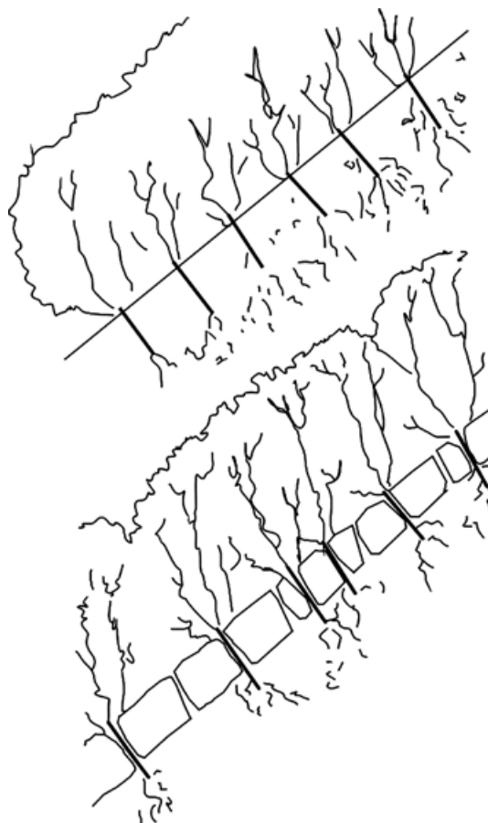
Rys. 65. Skarpa umocniona zrzezami wierzbowymi: a) na skarpie, b) w szczelinach bruku układanego na sucho [Begemann i Schiechtel 1999]
