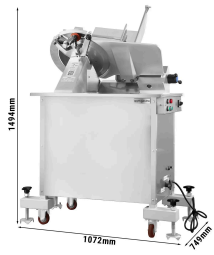
Automatický krájač Hendi - 750 wattov, nôž Ø 360 mm
