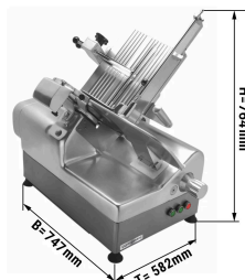
Automatický krájač Hendi - 370 wattov, nôž Ø 320 mm
