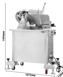
Automatický krájač Hendi - 750 wattov, nôž Ø 360 mm
