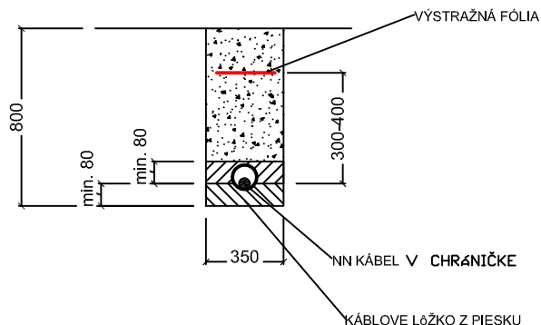
REZ 2 - 2 (VOLNÝ TERÉN)
