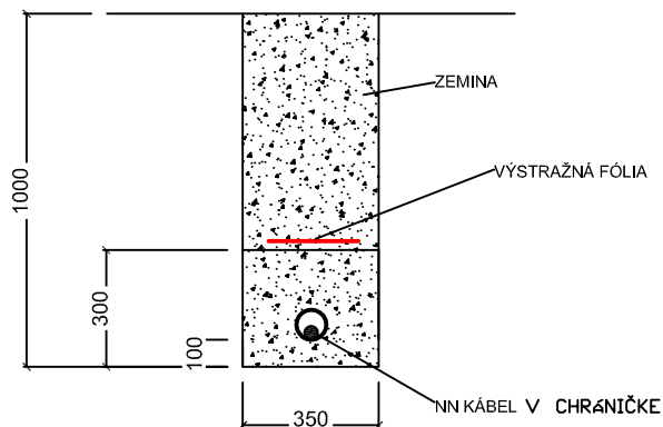
REZ 1 - 1 (KRIŽOVANIE S VOZOVKOU)
