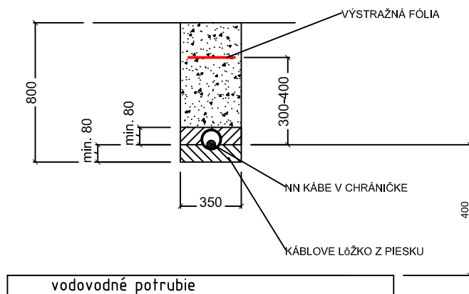
REZ 3 - 3 (KRIŽOVANIE S VODOU)
