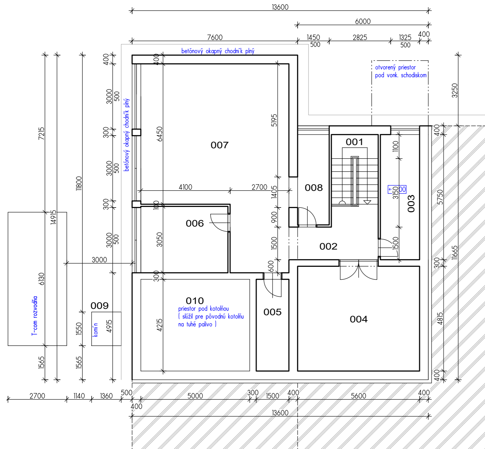
PÔDORYS SUTERÉNU - PÔVODNÝ STAV
