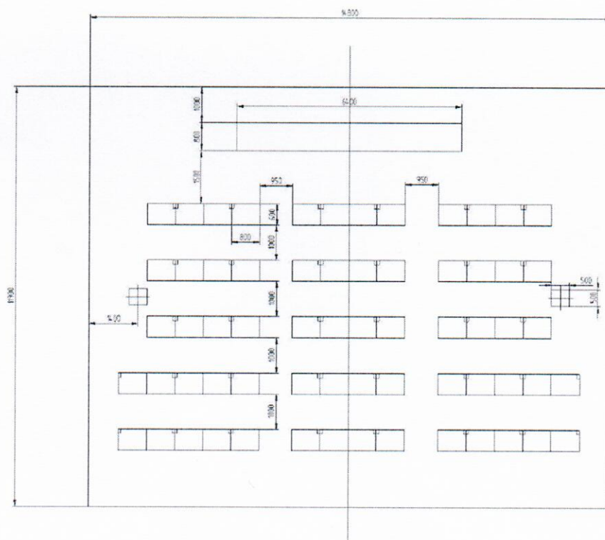
Schéma rozmiestnenia kongresových stolov a zástrčiek.
