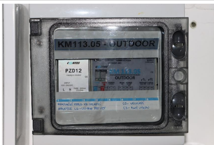
Pohled na rozvaděč s jističi pro VZT umístěný vedle rozvaděče MaR.
