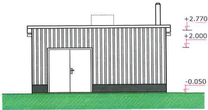
čelný pohľad
