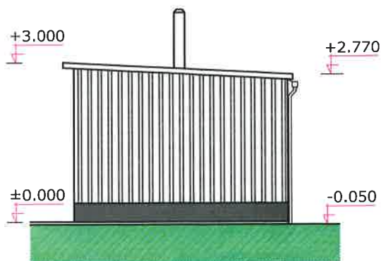
bočný pohľad
