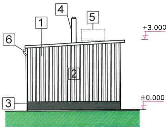
bočný pohľad
