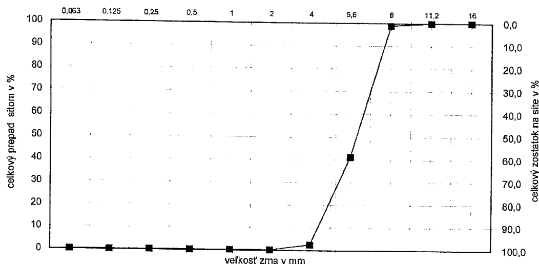
Grafické znázornenie zrnitosti kameniva
