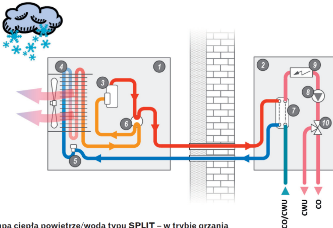
Rysunek 8 Powietrzna pompa ciepła typu split
