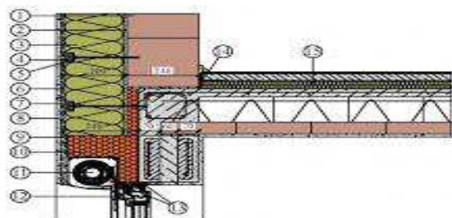
Použitie tepelnej izolácie KNAUF INSULATION v zatepľovacom systéme ETICS - nadpráhové okna/dvere s vonkajšou izoláciou - s tepelne izolovaným prvkom VARIO
