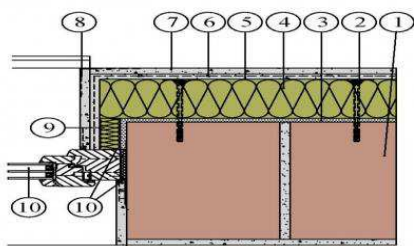
Použitie tepelnej izolácie KNAUF INSULATION v zatepľovacom systéme ETICS - detail u ostenia
