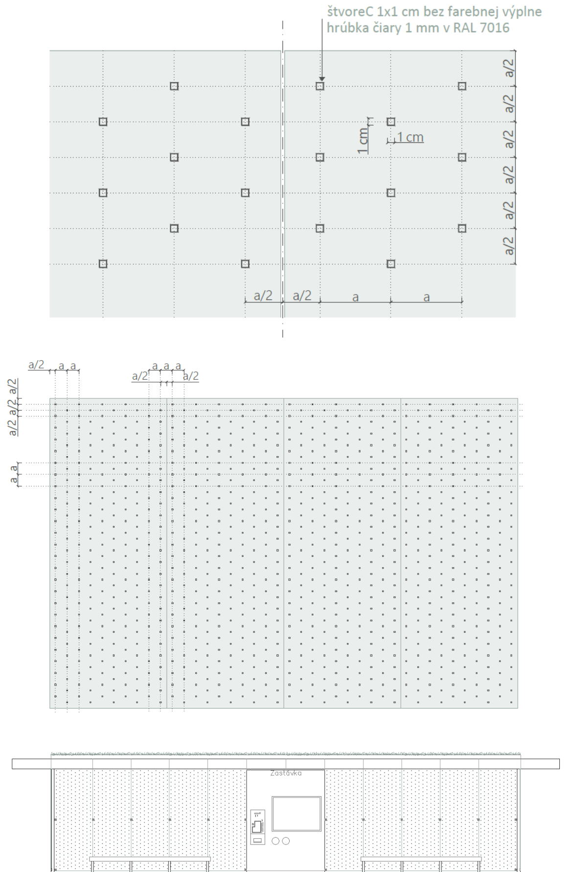
Obrázok 79_Vzor sieťotlače na sklenených stenách prístrešku na električkových zastávkach
