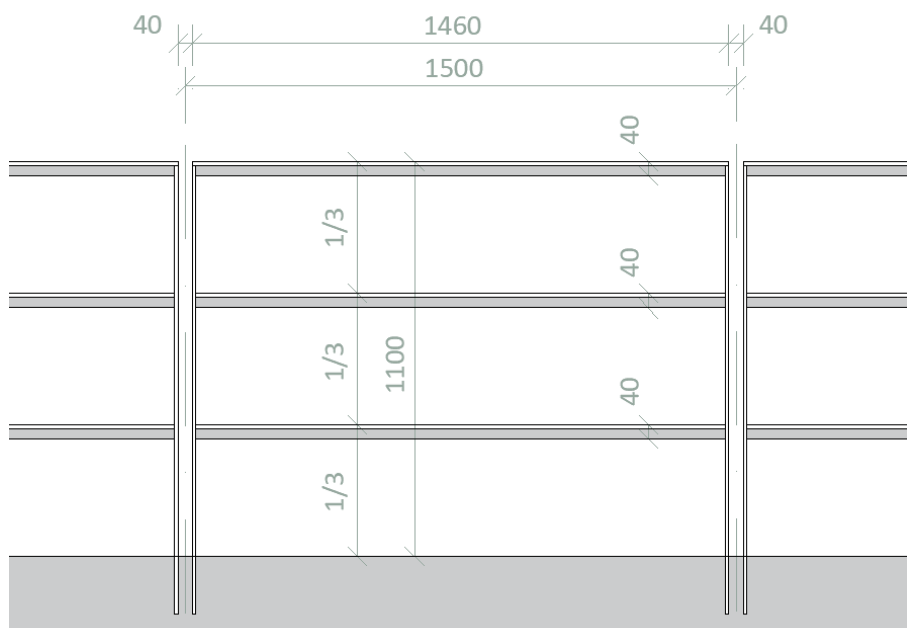
Obrázok 179_ Rozmery segmentu dizajnového dopravno-bezpečnostného zábradlia so šírkou 1460 mm
