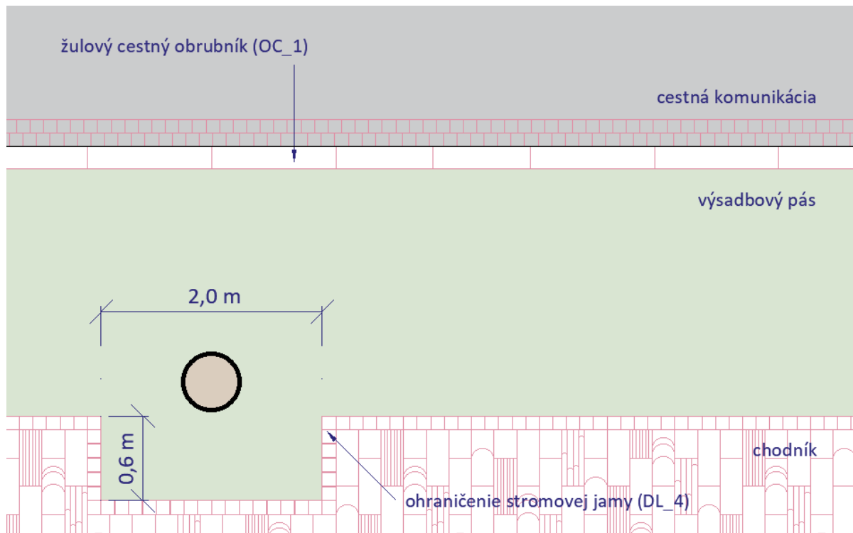
Obrázok 35_Stromová jama na Záhradníckej ulici
