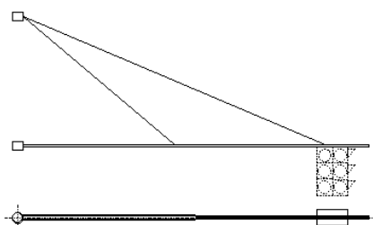
V10 dĺžka 8,0 m (orientačne) s kotviacim prvkom K2
