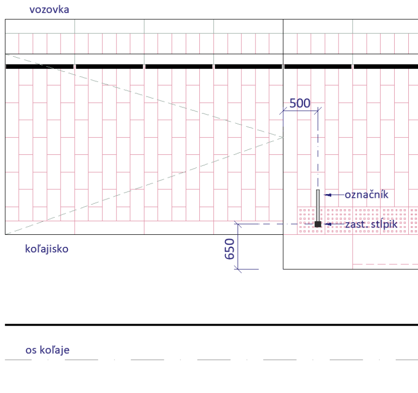
Obrázok 97_Pôdorysná schéma štandardného umiestnenia označníka na nástupišti
