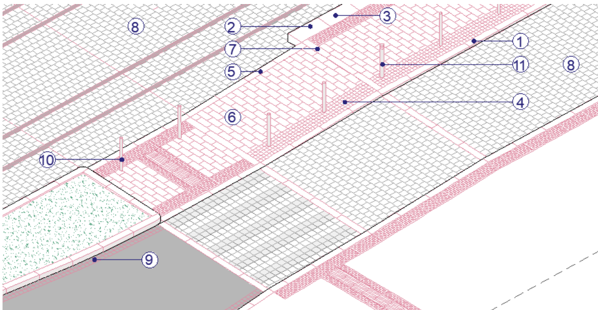
Obrázok 51_Dlažobné prvky na zastávke Krížna (koniec nástupišťa smer Centrum)
