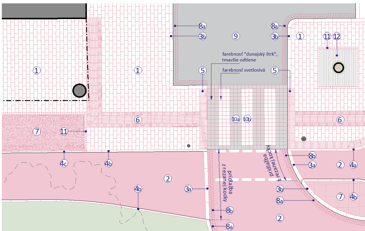
Obrázok 166_Materiálové riešenie povrchov v križovatke Krížna – Májkova (prieťah pre chodcov cez Májkovu ulicu)
