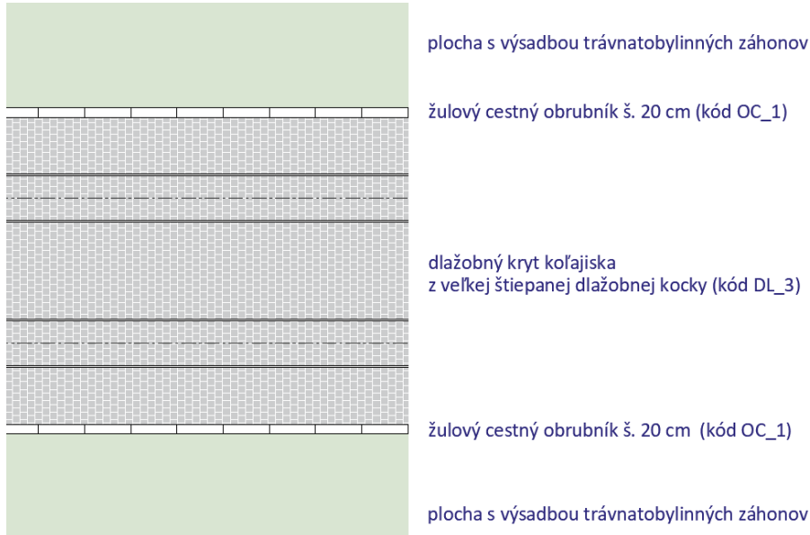
Obrázok 143_Pôdorysná schéma koľajiska – dlažobný kryt na Odborárskom námestí (táto schéma nenahrádza kladačský plán)
