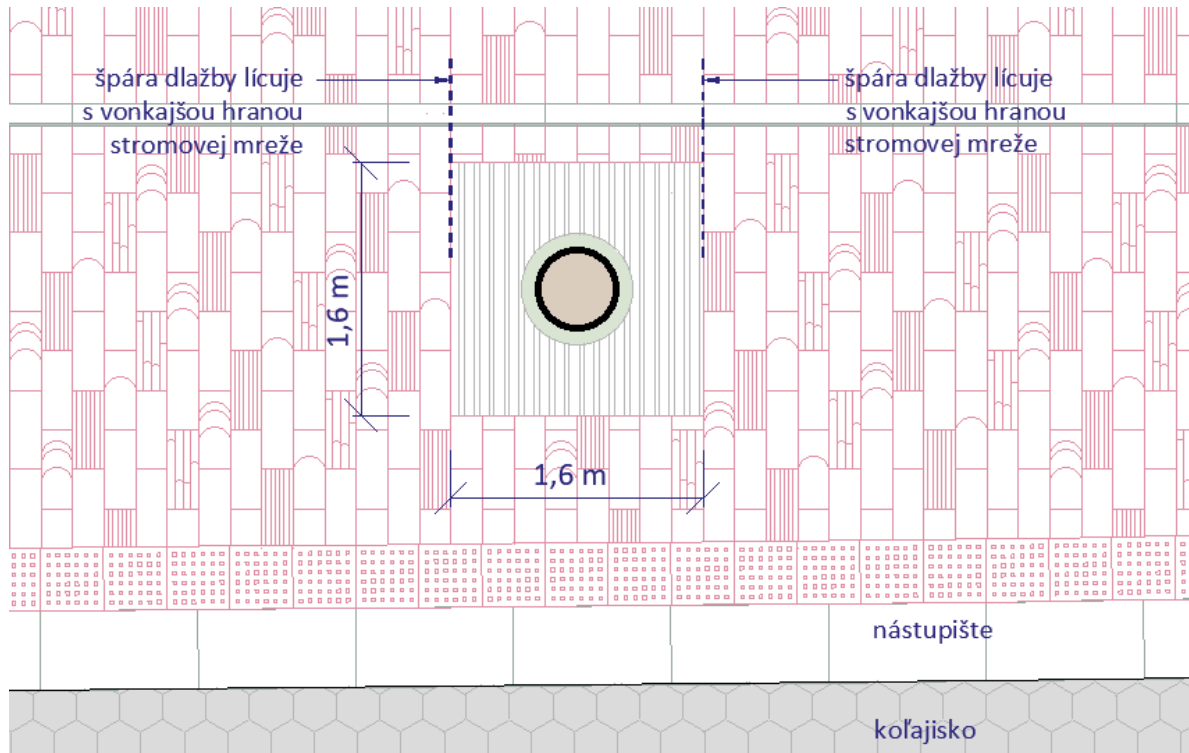
Obrázok 42_Stromové mreže pred areálom Saleziánov dona Bosca
