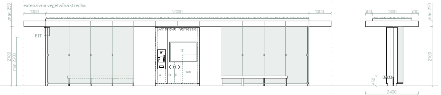
pohľad čelný
