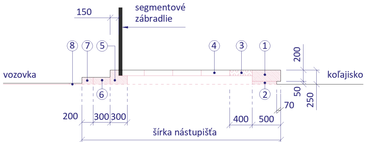
Obrázok 53_Priečny rez obojstranným nástupišťom v mieste lemovacieho múrika
