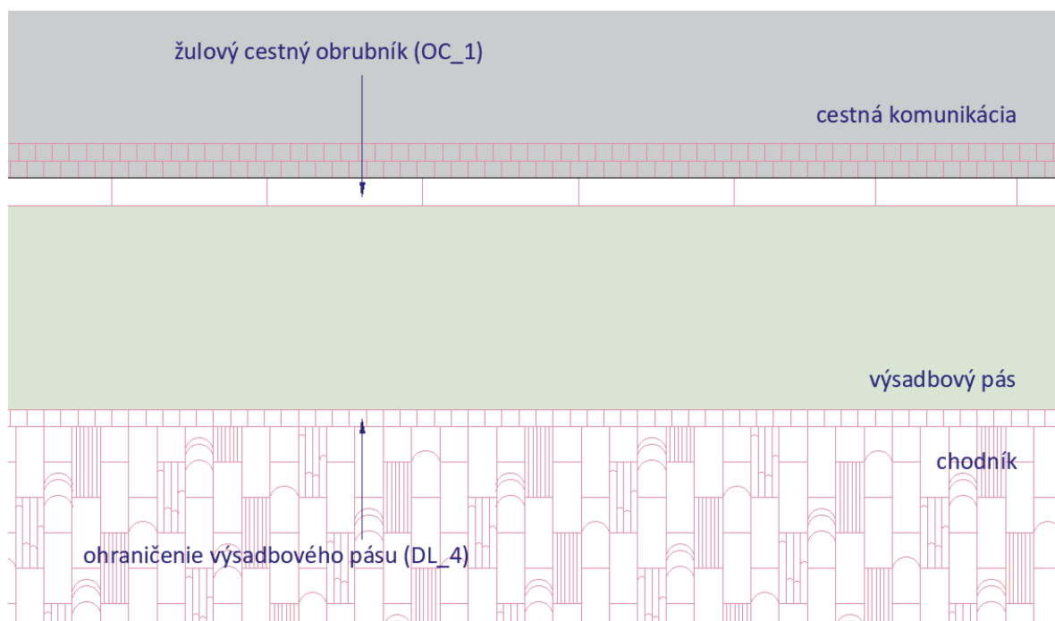
Obrázok 24_Príklad ohraničenia výsadbového pásu na Trnavskom mýte, pozdĺž cestnej komunikácie Krížna-smer Vajnorská
