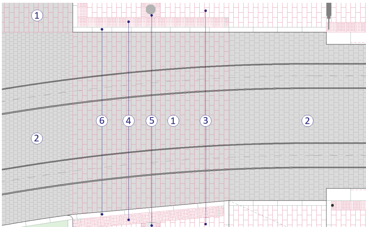
Obrázok 149_Priechod pre chodcov v rámci zastávky Americké námestie
