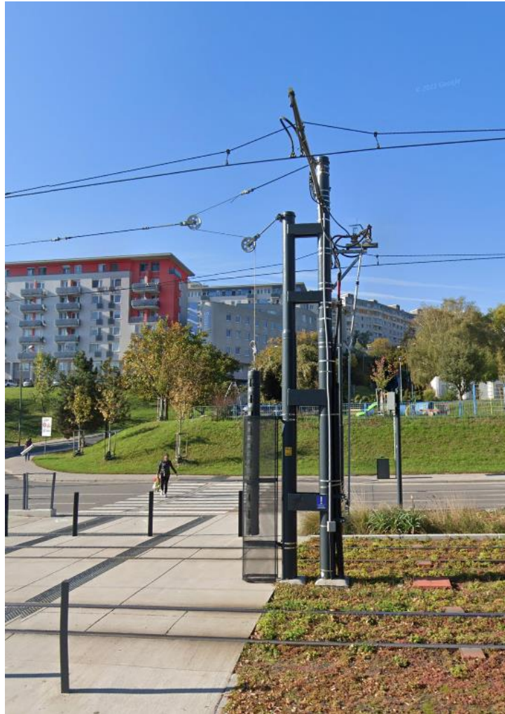
Obrázok 160_Príklad nežiadúceho riešenia vyvažovania trakčného stožiara
