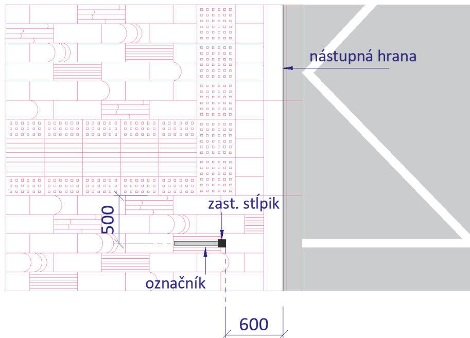
Schéma 129_Pôdorysná schéma preferovaného umiestnenia označníka na nástupišti
