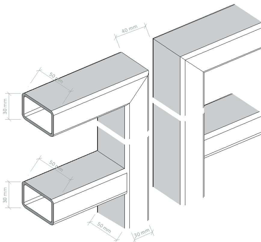
Obrázok 183_Detail napojenia vertikálnej a horizontálnej časti štandardného dopravno-bezpečnostného zábradlia
