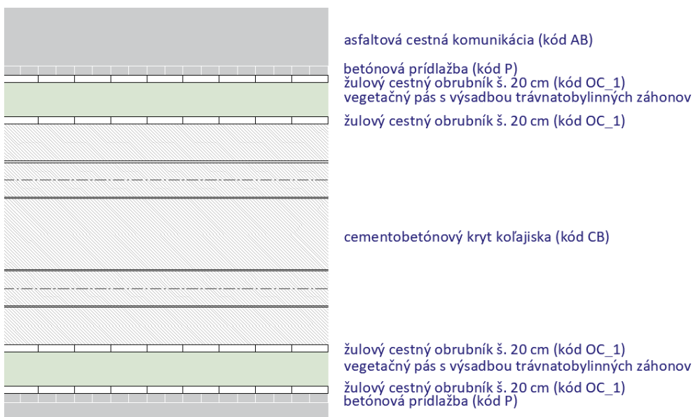
Obrázok 146_Pôdorysná schéma koľajiska – cementobetónový kryt (táto schéma nenahrádza kladačský plán)
