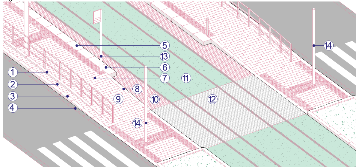
Obrázok 63_Dlažbobné a zastávkové prvky na zastávke Súmračná (začiatok nástupištia smer Astronomická)
