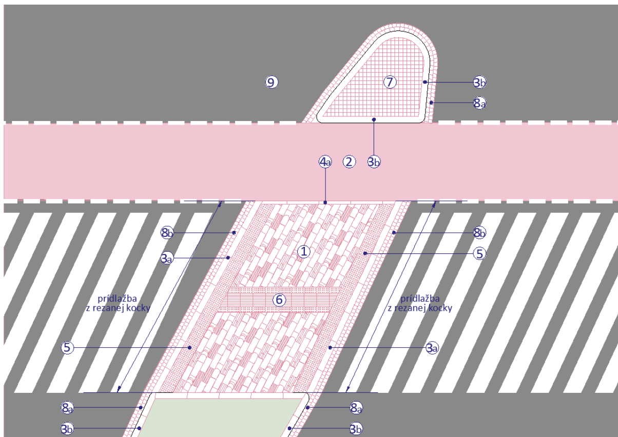
Obrázok 170_Materiálové riešenie povrchov na ostrovčeku v križovatke Krížna – Legionárska
