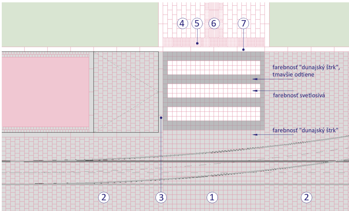
Obrázok 152_Priechod pre chodcov mimo zastávky – Krížna ulica
