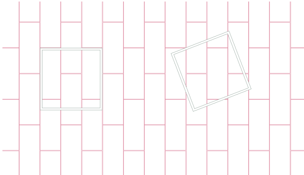
Obrázok 193_Kladenie dlažby v mieste zadlážďovacích poklopov
