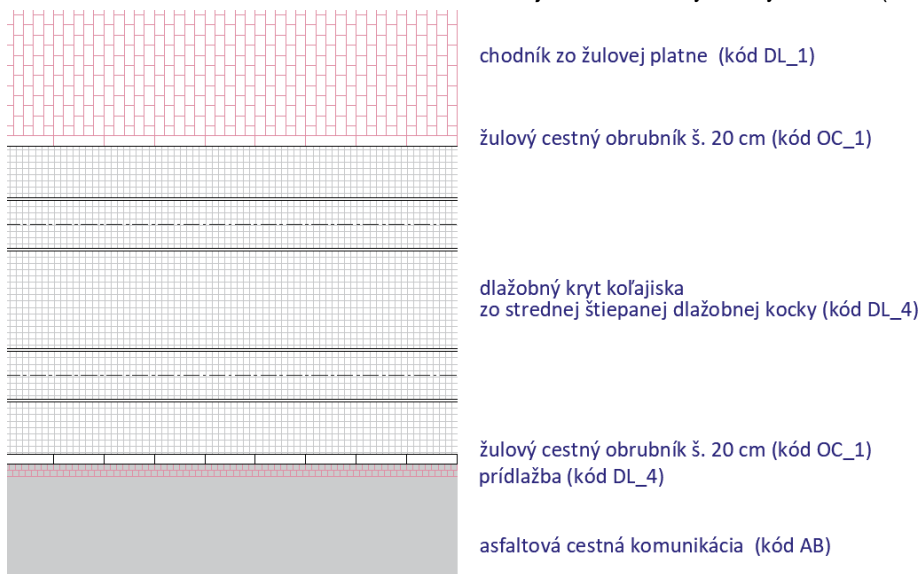
Obrázok 142_Pôdorysná schéma koľajiska – dlažobný kryt na Americkom námestí (táto schéma nenahrádza kladačský plán)
