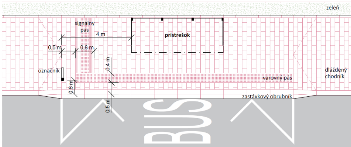
Obrázok 139_Pôdorysná schéma usporiadania zastávky na dláždenom chodníku
