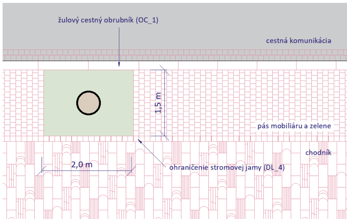
Obrázok 33_Stromová jama na Krížnej ulici v úseku 2
