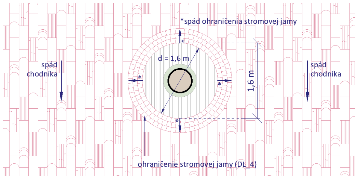
Obrázok 38_Stromové mreže na Trnavskom mýte
