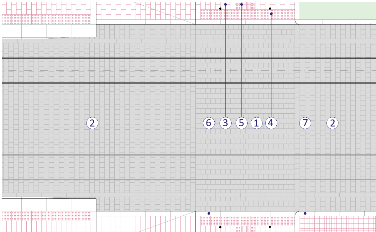
Obrázok 150_Priechod pre chodcov v rámci zastávky Krížna
