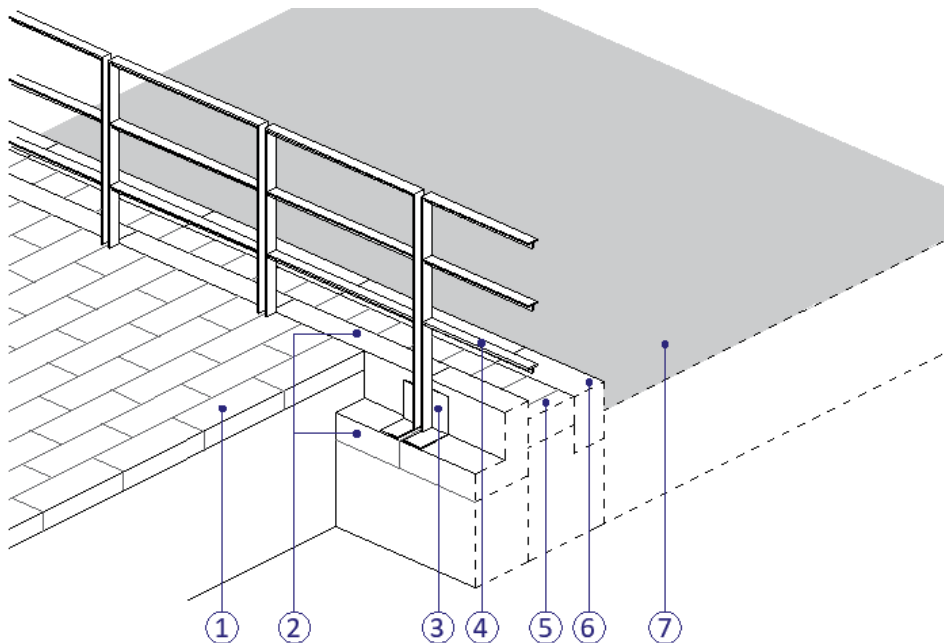
Obrázok 85_Schéma kotvenia zábradlia pod povrchom dlažby
