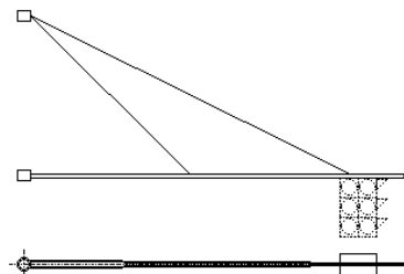
V9 dĺžka 7,0 m (orientačne) s kotviacim prvkom K2
