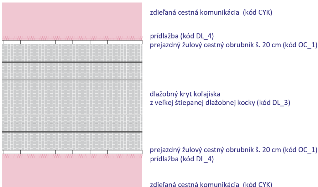
Obrázok 144_Pôdorysná schéma koľajiska – dlažobný kryt na Križnej ulici (táto schéma nenahrádza kladačský plán)
