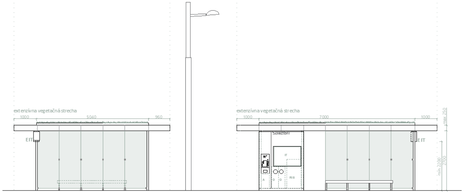
pohľad čelný
