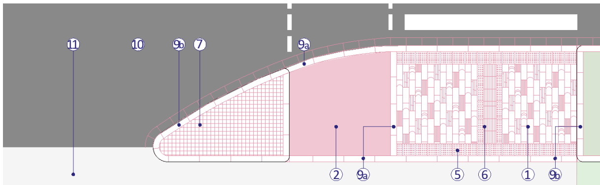
Obrázok 172_Materiálové riešenie povrchov v križovatke Ružinovská – Tomášikova – vyčkávacia plocha pre chodcov a cyklistov medzi cestnou komunikáciou a koľajiskom
