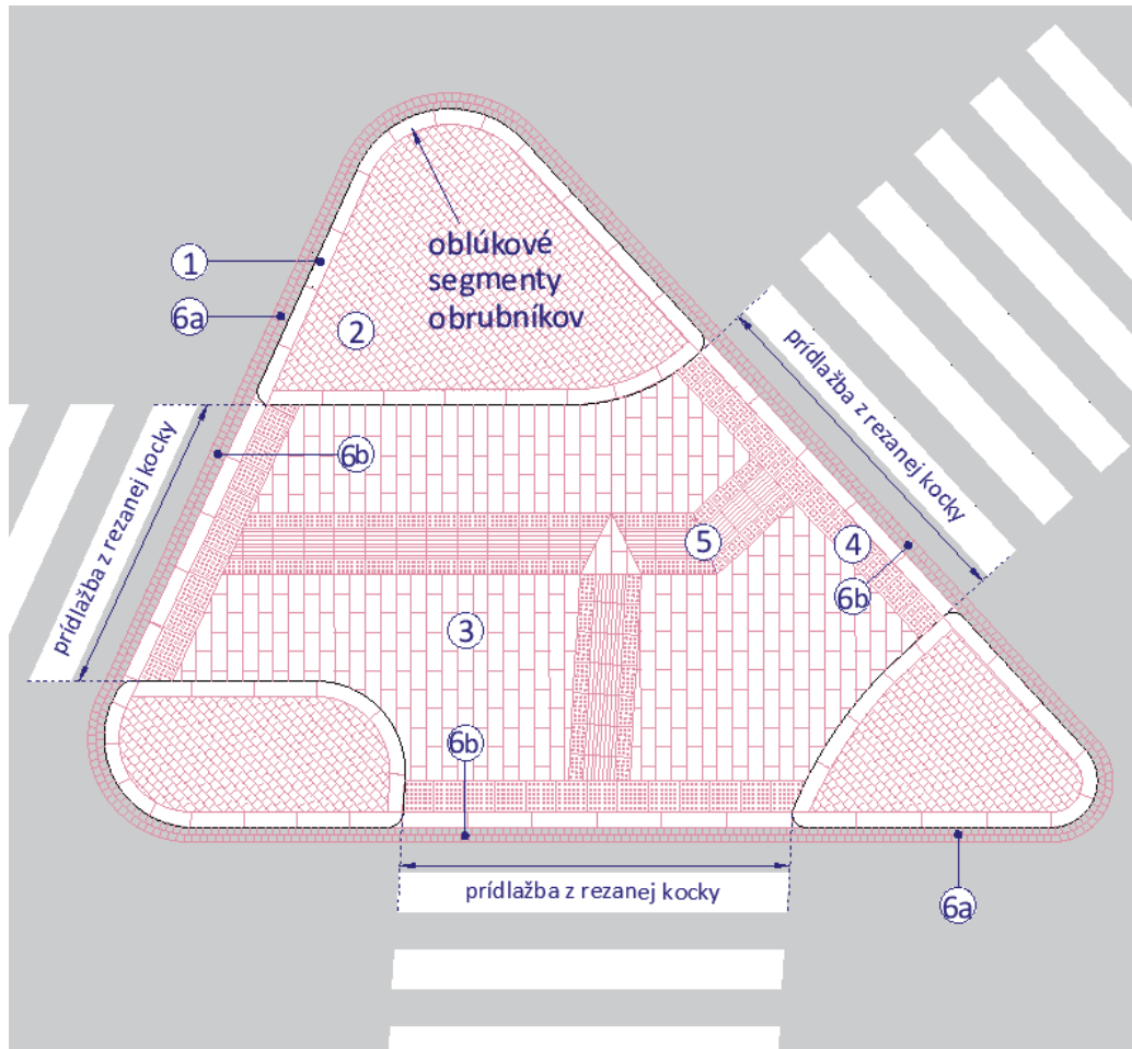
Obrázok 20_Příklad trojramenného ostrovčeka s priechodom pre chodcov v úseku 2 po km 2,55 (táto schéma nenahrádza kladačský plán)
