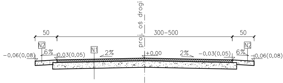
PRZEKRÓJ ODCINEK PROSTY
