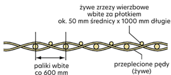
Rys. 75. Schemat płotki plecionego [Krukowski 2006]
