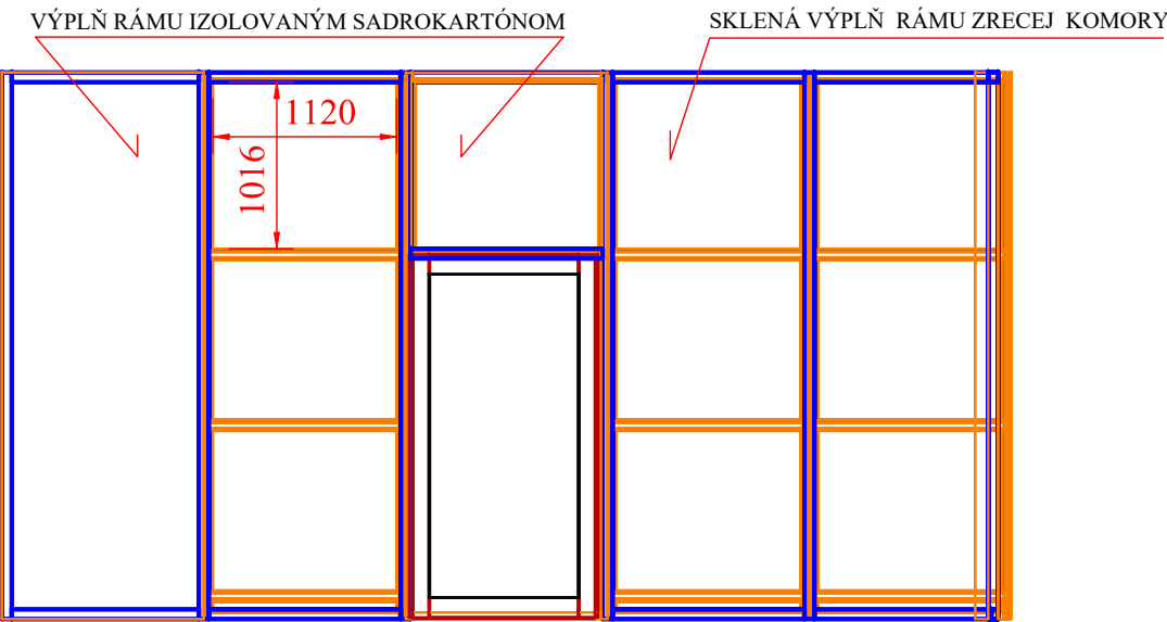
ZVAROVANÝ KOVOVÝ RÁM ZRECEJ KOMORY
