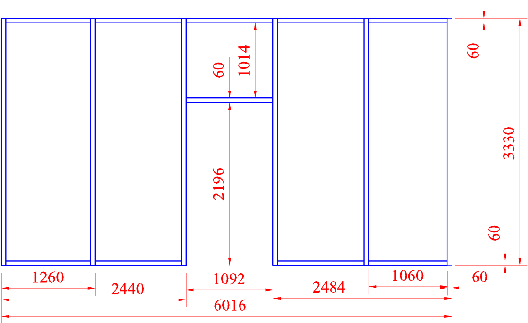
ZVAROVANÝ KOVOVÝ RÁM ZRECEJ KOMORY
