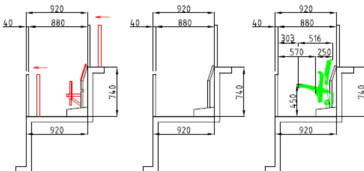
Úprava rámu existujúcej stolice u Tribúny A.
