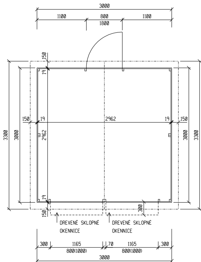
Pôdorys
