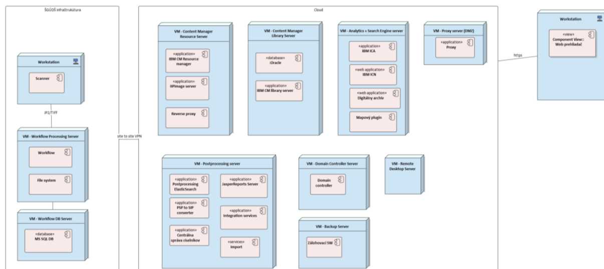
Obrázok 8 - Budúce riešenie v cloude
