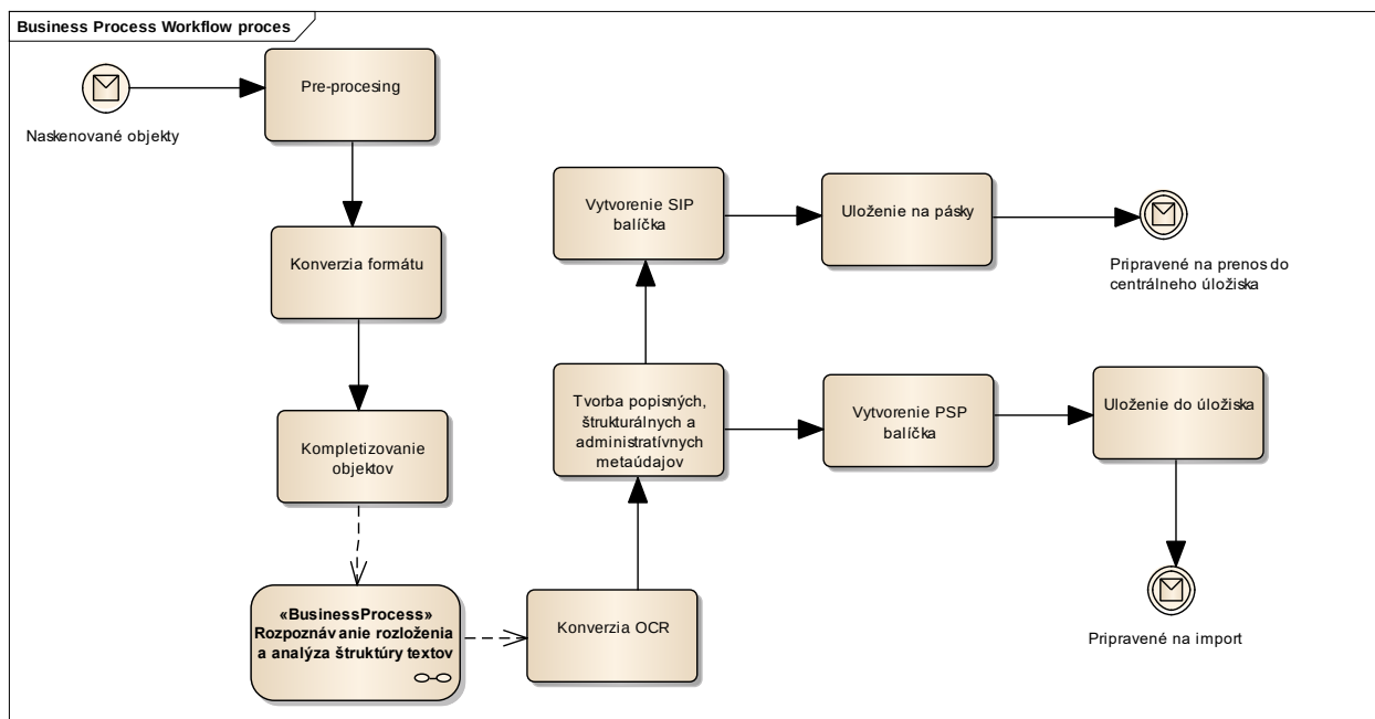
Obrázok 4 Workflow proces skenovaných dokumentov
