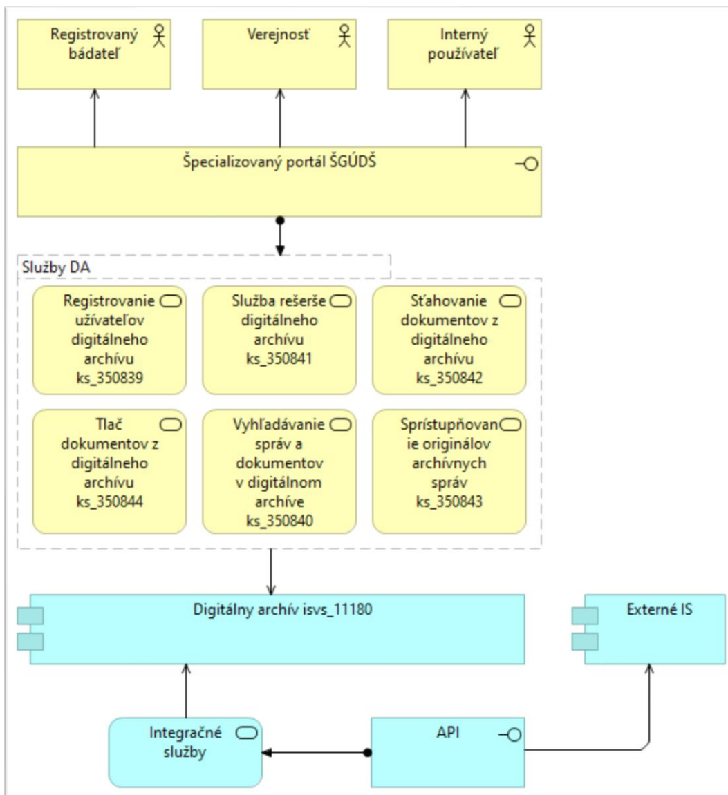
Obrázok 1 Biznis architektúra Digitálneho archívu AS IS
