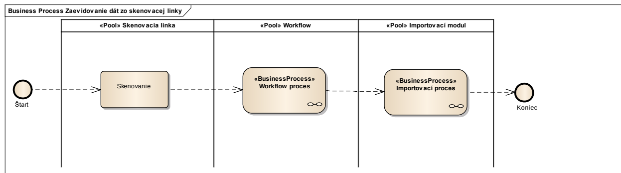
Obrázok 3 Hlavný proces – zaevidovanie dát zo skenovacej linky
