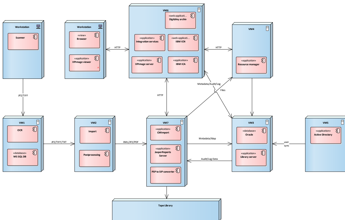
Obrázok 6 Model nasadenia Digitálneho archívu vo virtualizovanej infraštruktúre
