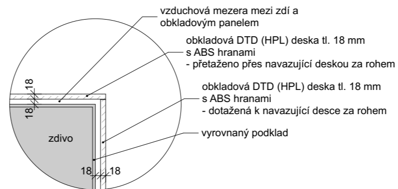
Detail návaznosti obkladových panelů v rohu a na nároží stěny- půdorys
