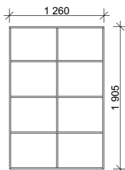
Nárys bez dvířek
