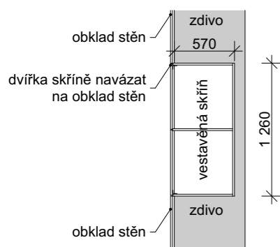
Půdorys
