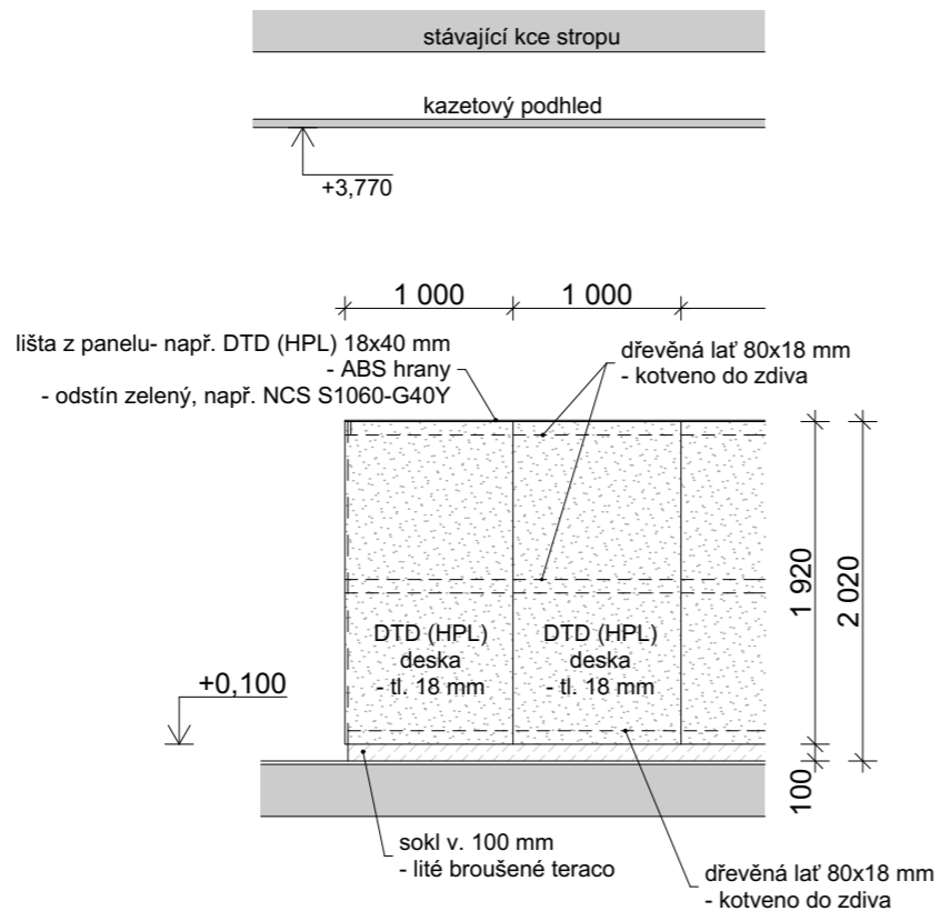
Charakteristický pohled
