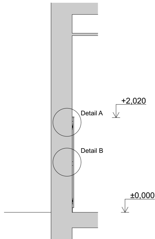
Charakteristický řez
