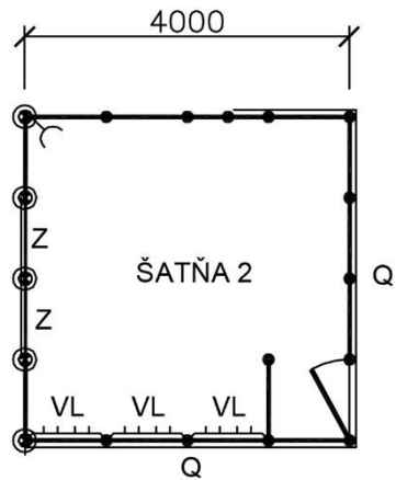
ŠATŇA 2 - SAMOSTATNE STOJACA
