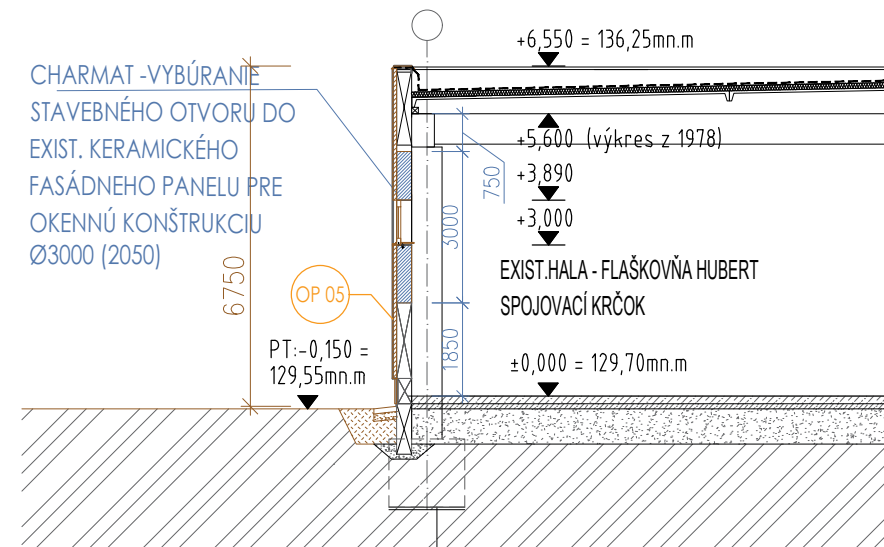
REZ 1-1 - Hubert fľaškovňa - spojovací krčok
