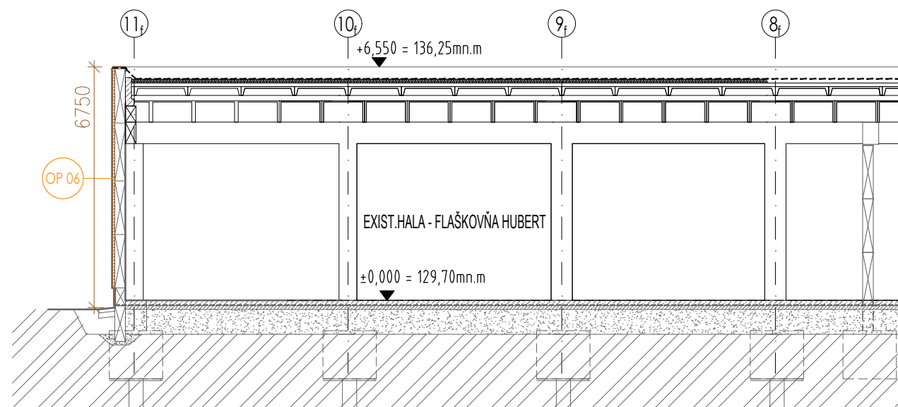
REZ 3-3 - Hubert fľaškovňa
