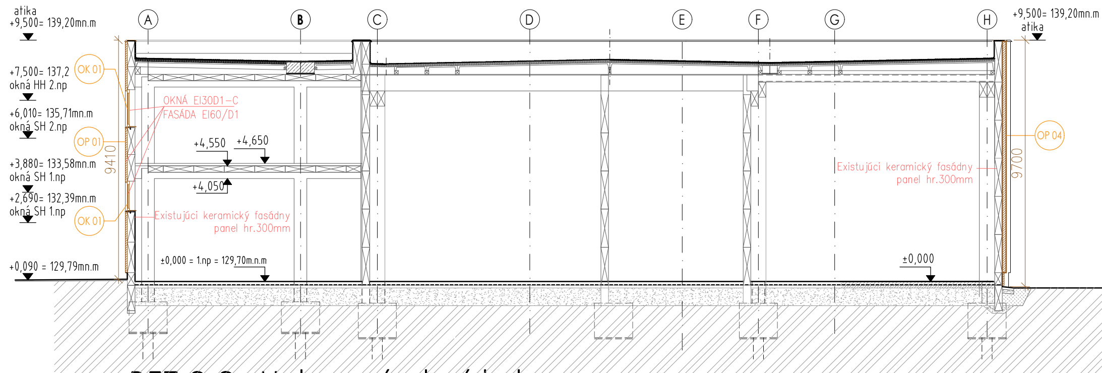
REZ C-C - Hubert výrobná hala
