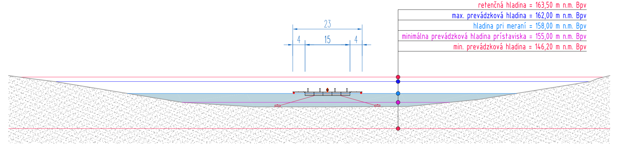
DNOVÝ PROFIL "A" M 1:750
