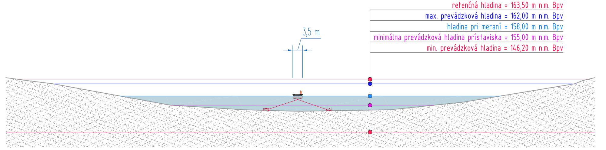
DNOVÝ PROFIL "B" M 1:750
