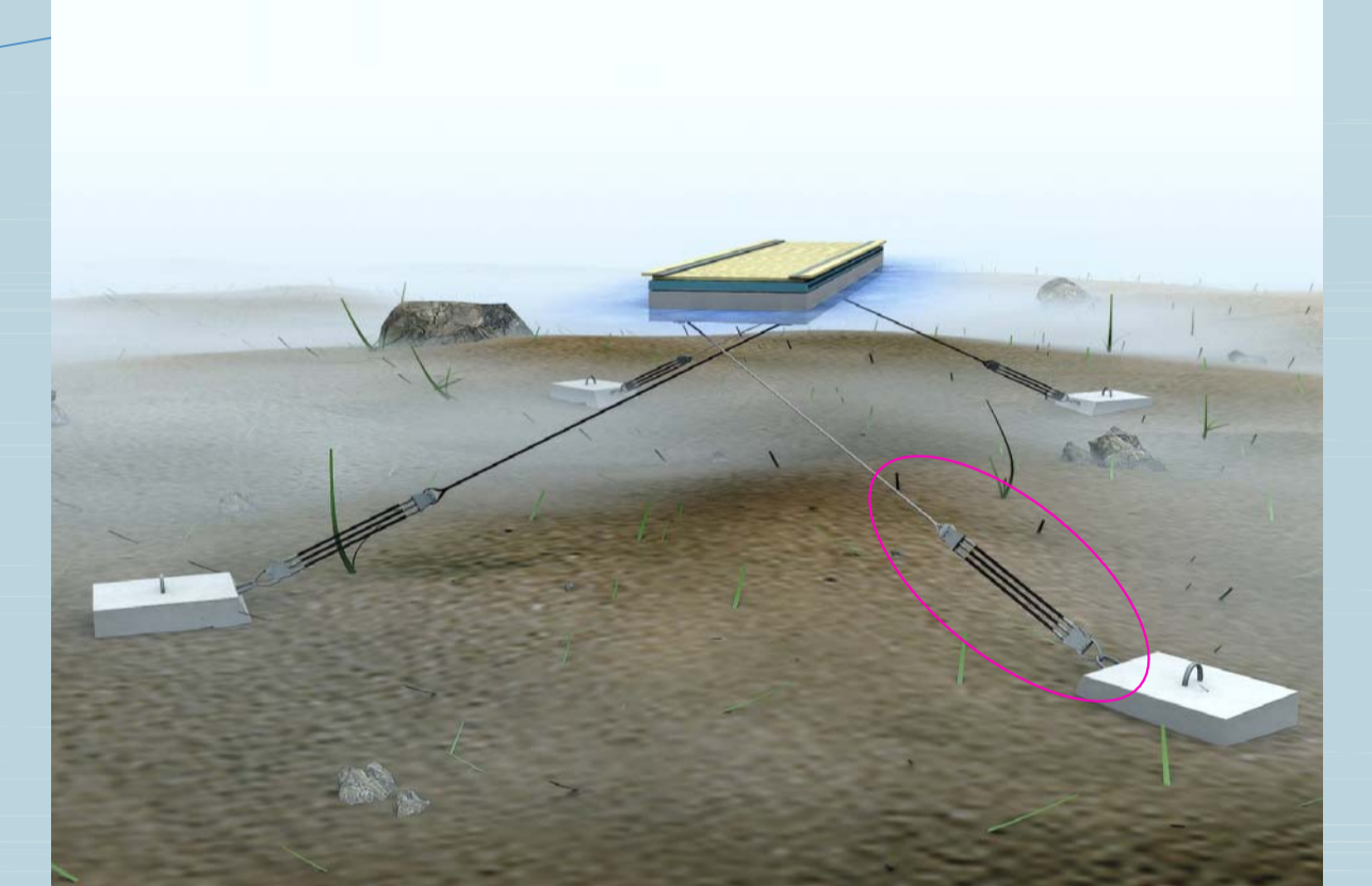
Príklad pružného kotviaceho systému s elastomérovými prvkami.
