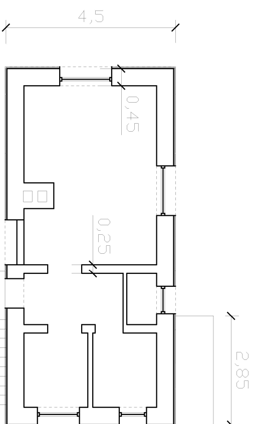
RZUT PARTERU
