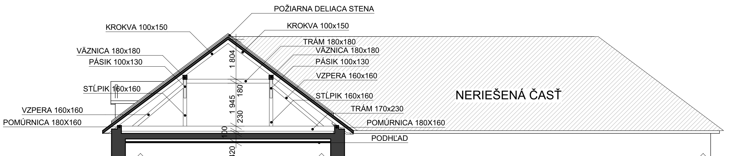
PRIEČNY REZ A-A M 1:100
