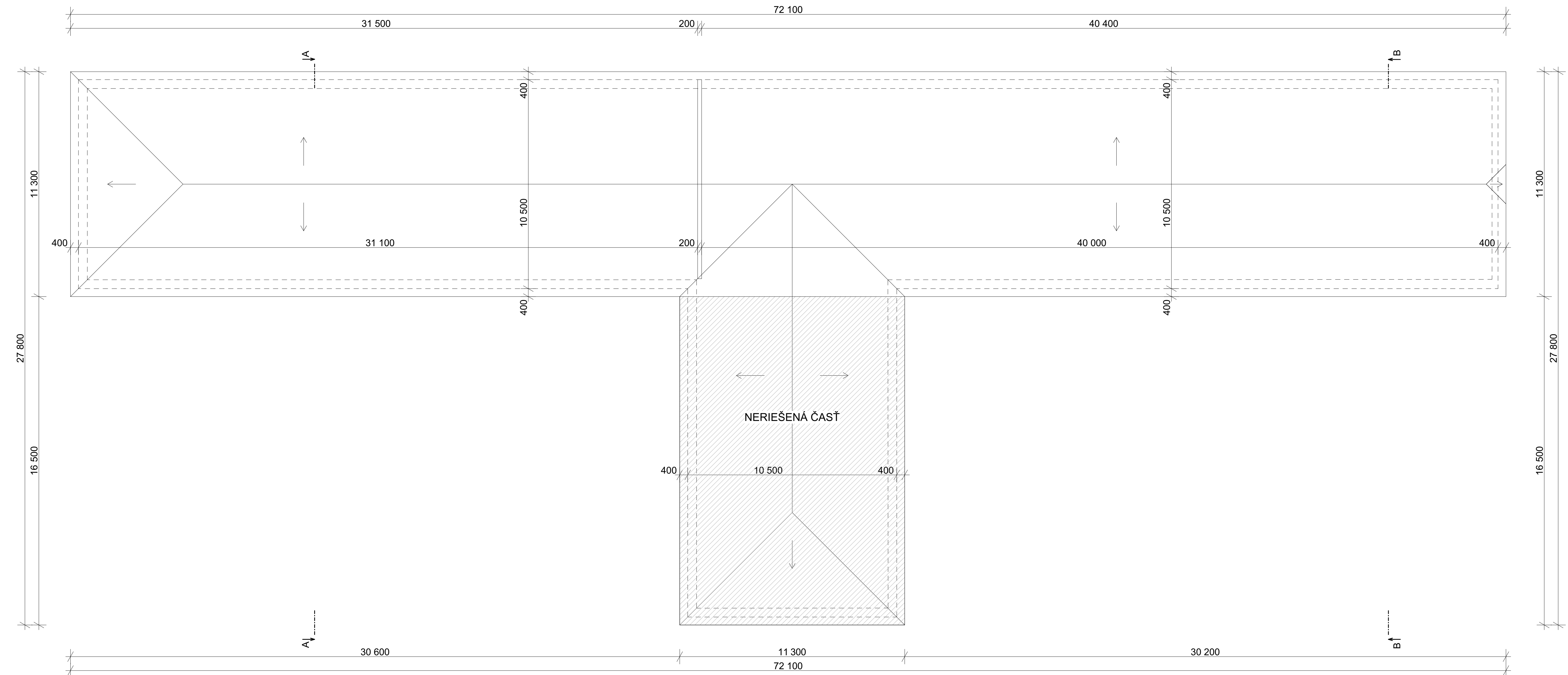
PÔDORYS STRECHY M 1:100
