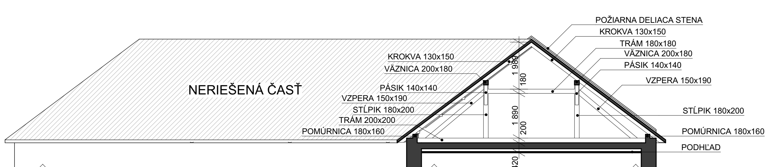
PRIEČNY REZ B-B M 1:100
