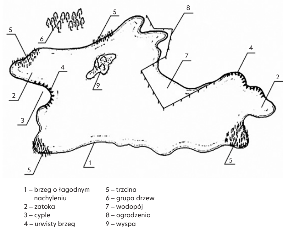
Rys. 11. Różnorodne ukształtowanie brzegów zbiornika [Żbikowski i Żelazo 1993]
