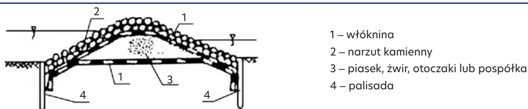
Rys. 43. Próg z piasku, żwiru lub otoczków umocnionych narzutem kamiennym na włókninie [Jędryka 2006]
