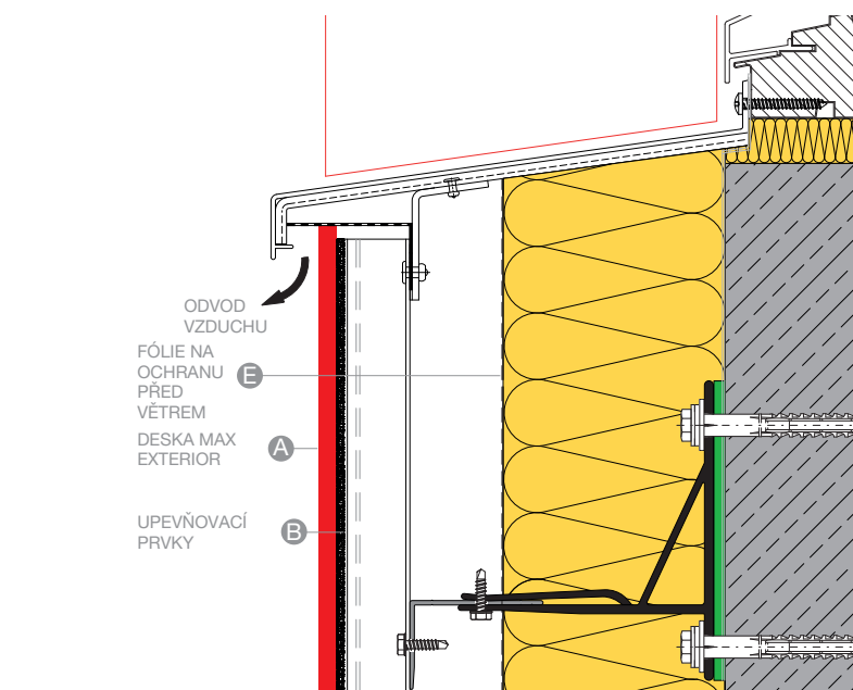
VODOROVNÁ SPÁRA A102
