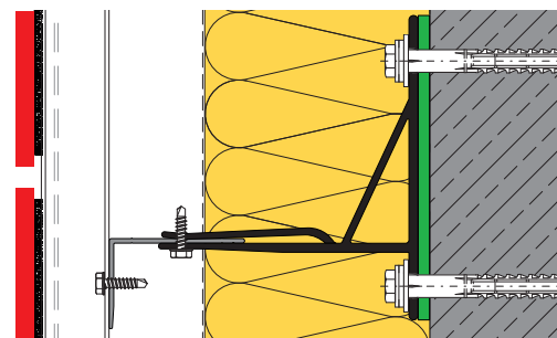
HORIZONTALNÍ SPÁRY A110
