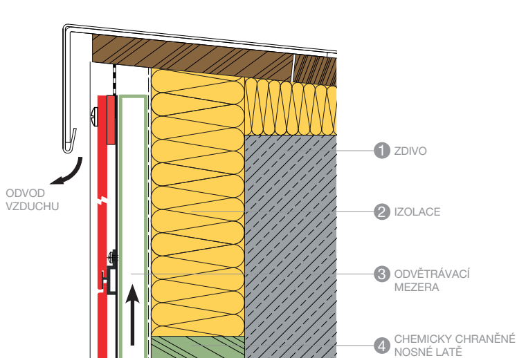
STŘEŠNÍ NAPOJENÍ - ATIKA A109
