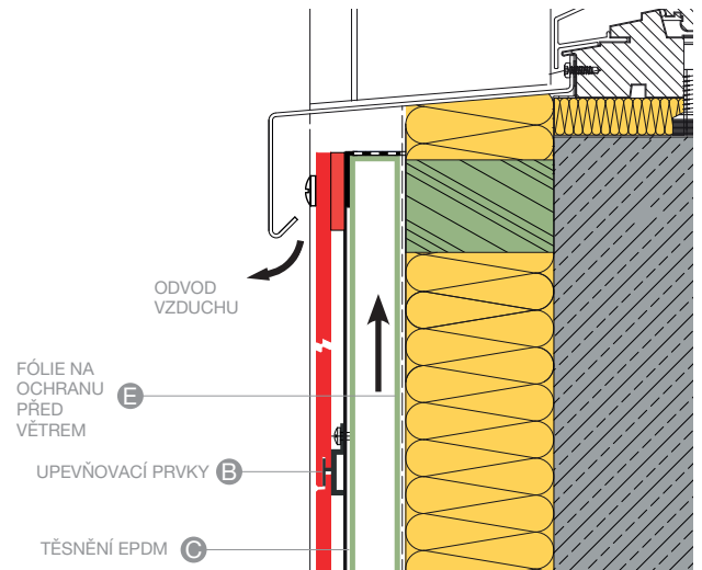
NAPOJENÍ OKENNÍHO PARAPETU A102
