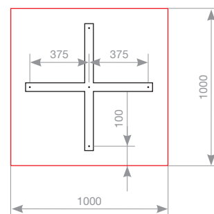
PŘÍKLAD STOLOVÉ DESKY-PŘESAHA
