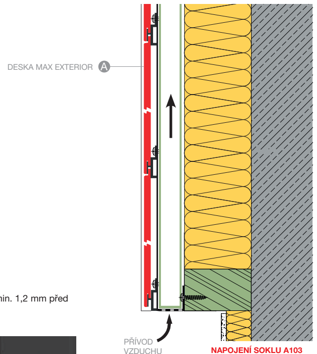
NAPOJENÍ SOKLU A103
