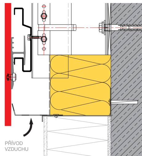
NAPOJENÍ NA PODEZDÍVKU A103
