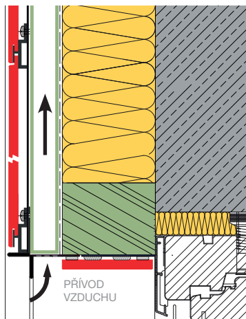
HORIZONTÁLNÍ SPÁRA A101
