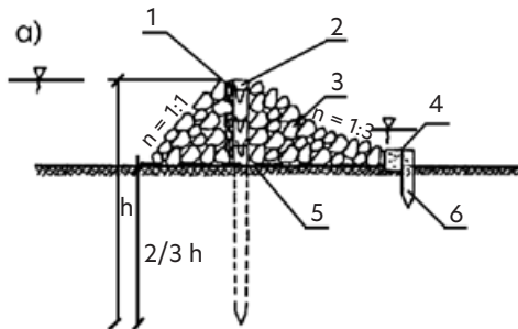
Rys. 42. Progi o konstrukcji mieszanej [Jędryka 2006]
