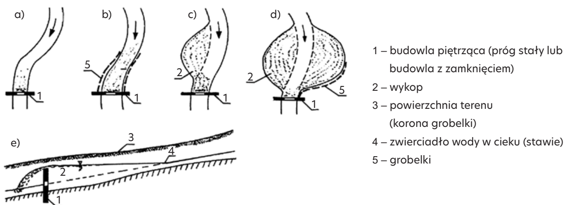
Rys. 15. Przykłady zwiększenia retencji koryt małych cieków naturalnych lub rowów: a) w obrębie istniejącego koryta, b) w granicach koryta rzeki z grobelkami, c, d) koryto cieków (rowu) poszerzone po jednej stronie/po obu stronach, e) profil podłużny cieków [Mioduszewski 2014]
