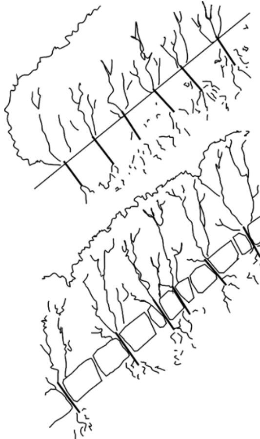
Rys. 65. Skarpa umocniona zrzezami wierzbowymi: a) na skarpie, b) w szczelinach bruku układanego na sucho [Begemann i Schiechl 1999]
