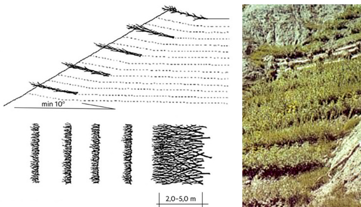
Rys. 66. i Fot. 64. Krzewiaste umocnienia tarasowe na skarpie/osuwisku [Begemann i Schiechtl 1999]
