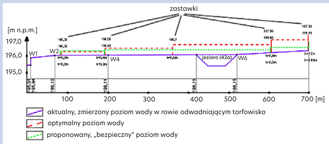
Rys. 23. Stopniowe podpiętrzanie wody na mokradle w ramach renaturyzacji prowadzonej przez Klub Przyrodników w rezerwacie „Jeziorka Chrościckie” (rys. P. Włodarczyk, na podstawie: Herbichowa i in. [2007])
