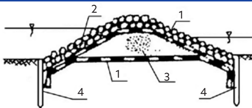
Rys. 43. Próg z piasku, żwiru lub otoczków umocnionych narzutem kamiennym na włókninie [Jędryka 2006]
