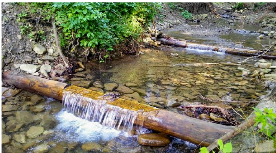
Fot. 42. Próg drewniany z przelewem z okrągłaków (fot. I. Biedroń [Biedroń 2018])
