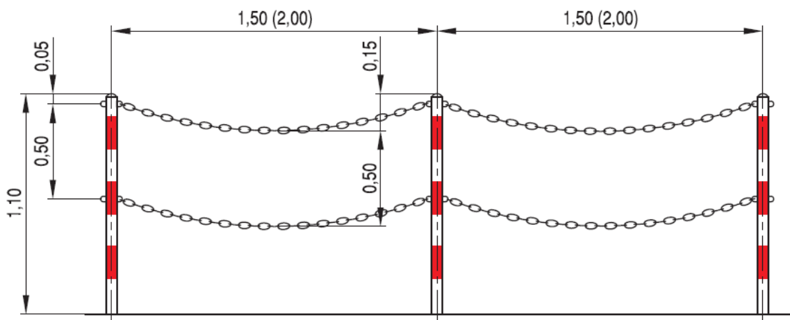
Rys. 6. Przykład ogrodzenia łańcuchowego U-12b [39]
