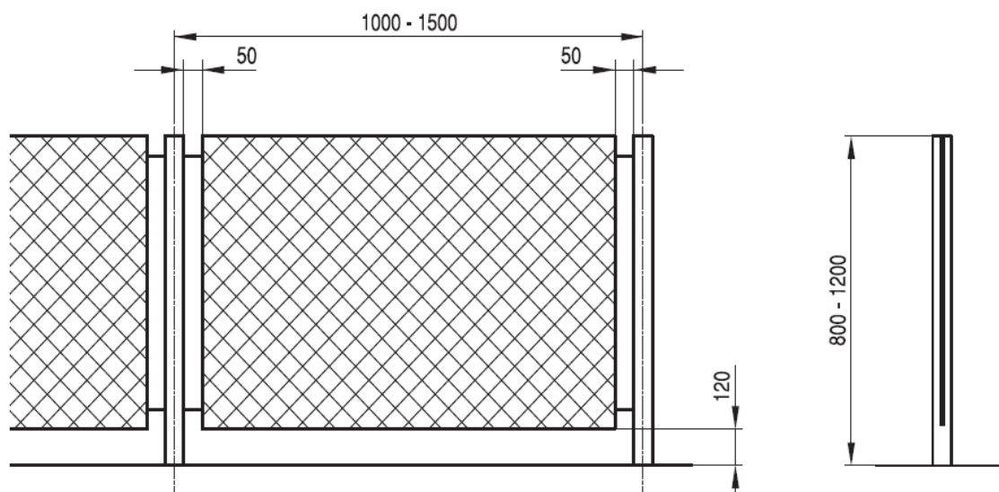
Rys. 5. Przykład ogrodzenia segmentowego U-12a [39]
