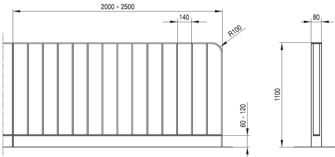
Rys. 4. Przykład balustrady U-11a [39]
