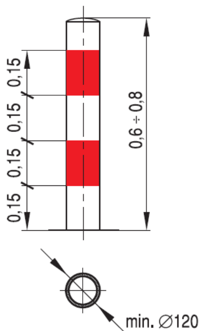
Rys. 7. Przykład słupka blokującego U-12e [39]
