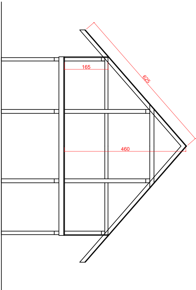
przekrój B-B
