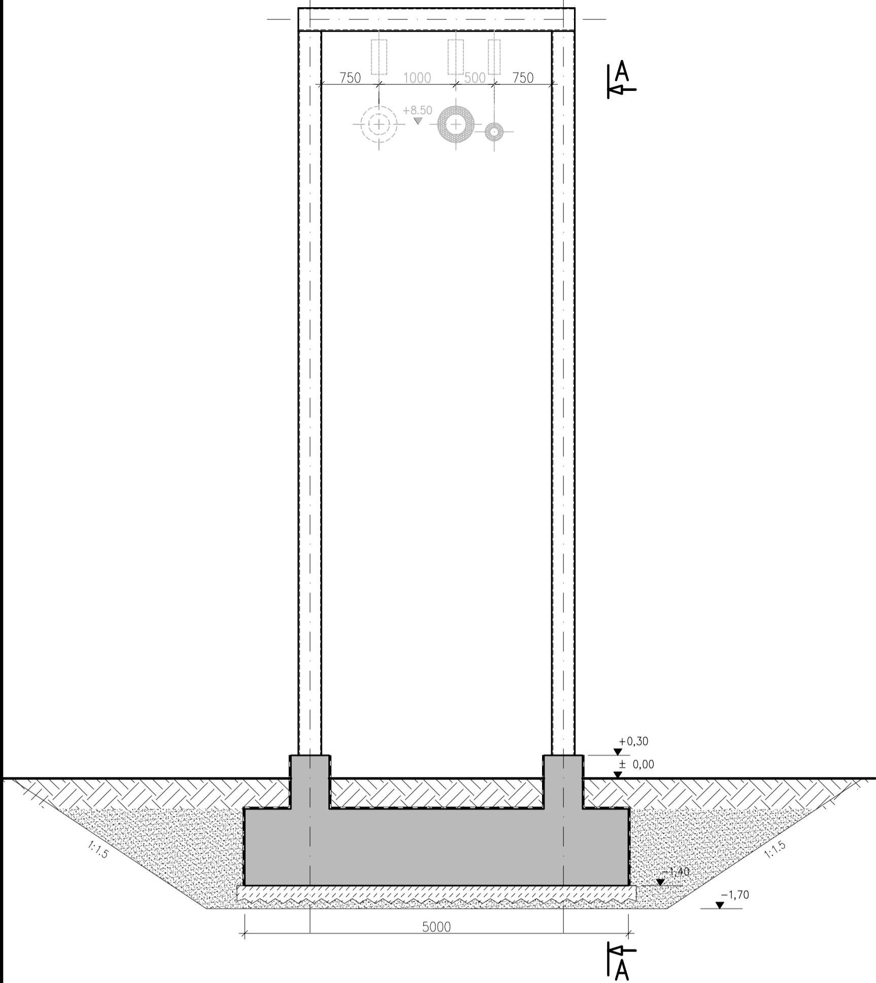
Przekrój B-B 1:50
