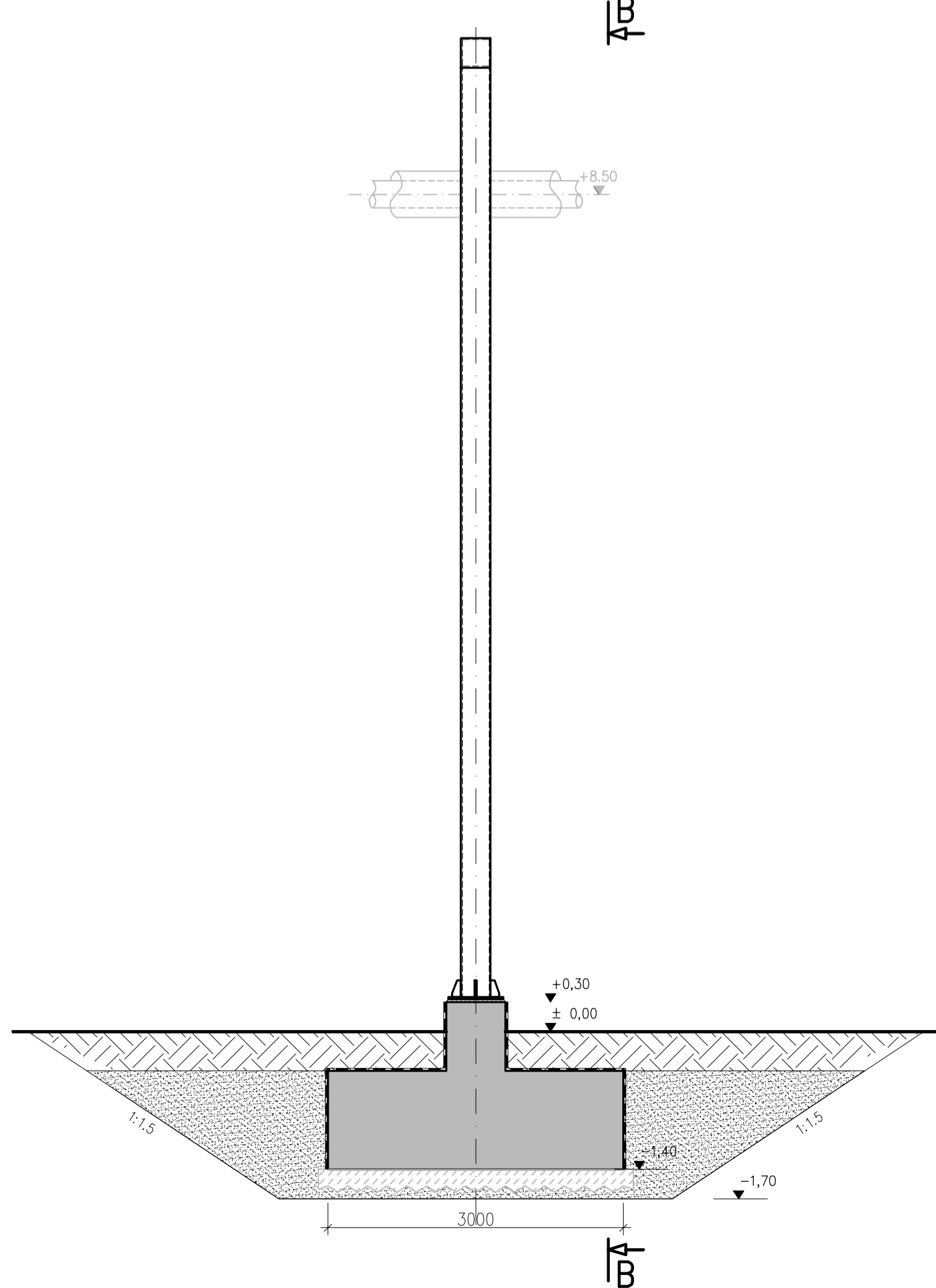
Przekrój A-A 1:50
