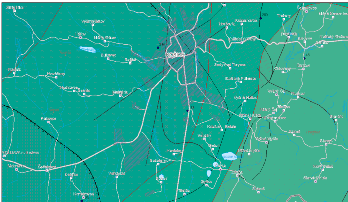
Obrázok 57: Geotermálna mapa 1000 m pod povrchom
