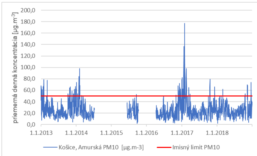
Obrázok 97: Priemerné denné koncentrácie PM 10 , stanica Amurská
