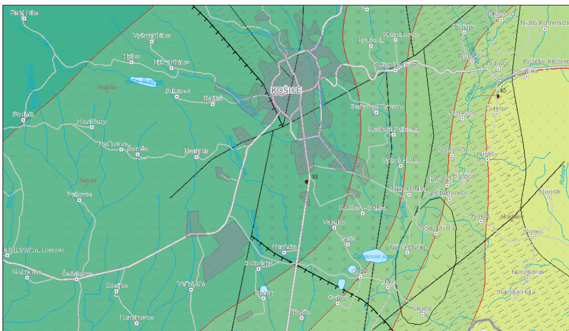
Obrázok 58: Geotermálna mapa 2000 m pod povrchom
