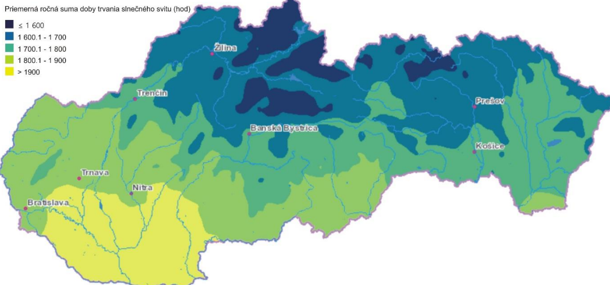
Obrázok 14: Priemerná ročná doba trvania slnečného svitu (1961 - 2010)
