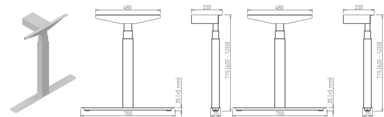
Rozmery stolovej podnože ELTIPLA 2
