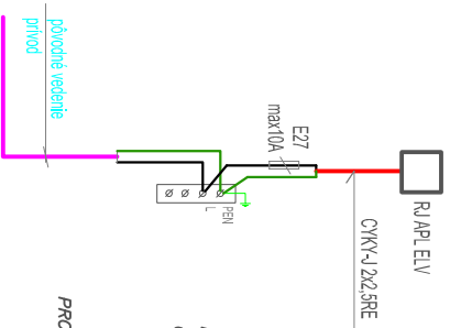
SCHEMA ZAPOJENIA NN ROZVODU
