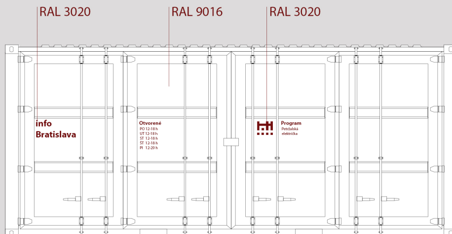
POHĽAD PREDNÝ M 1:50
