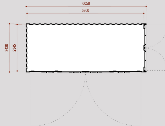
PÔDORYS M 1:100
