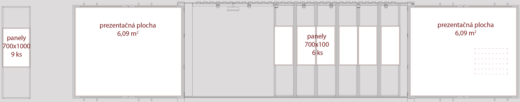
ČELNÝ POHĽAD M 1:50
