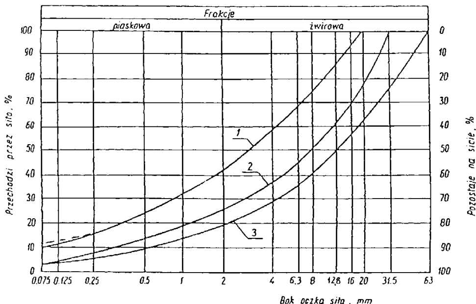
Rysunek 1. uziarnienia
