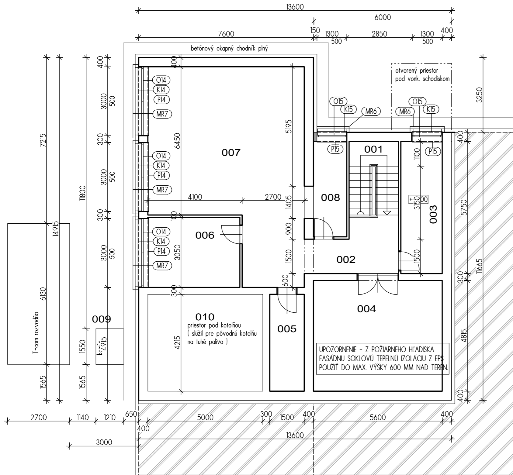
PÔDORYS SUTERÉNU - NAVRHOVANÝ STAV
