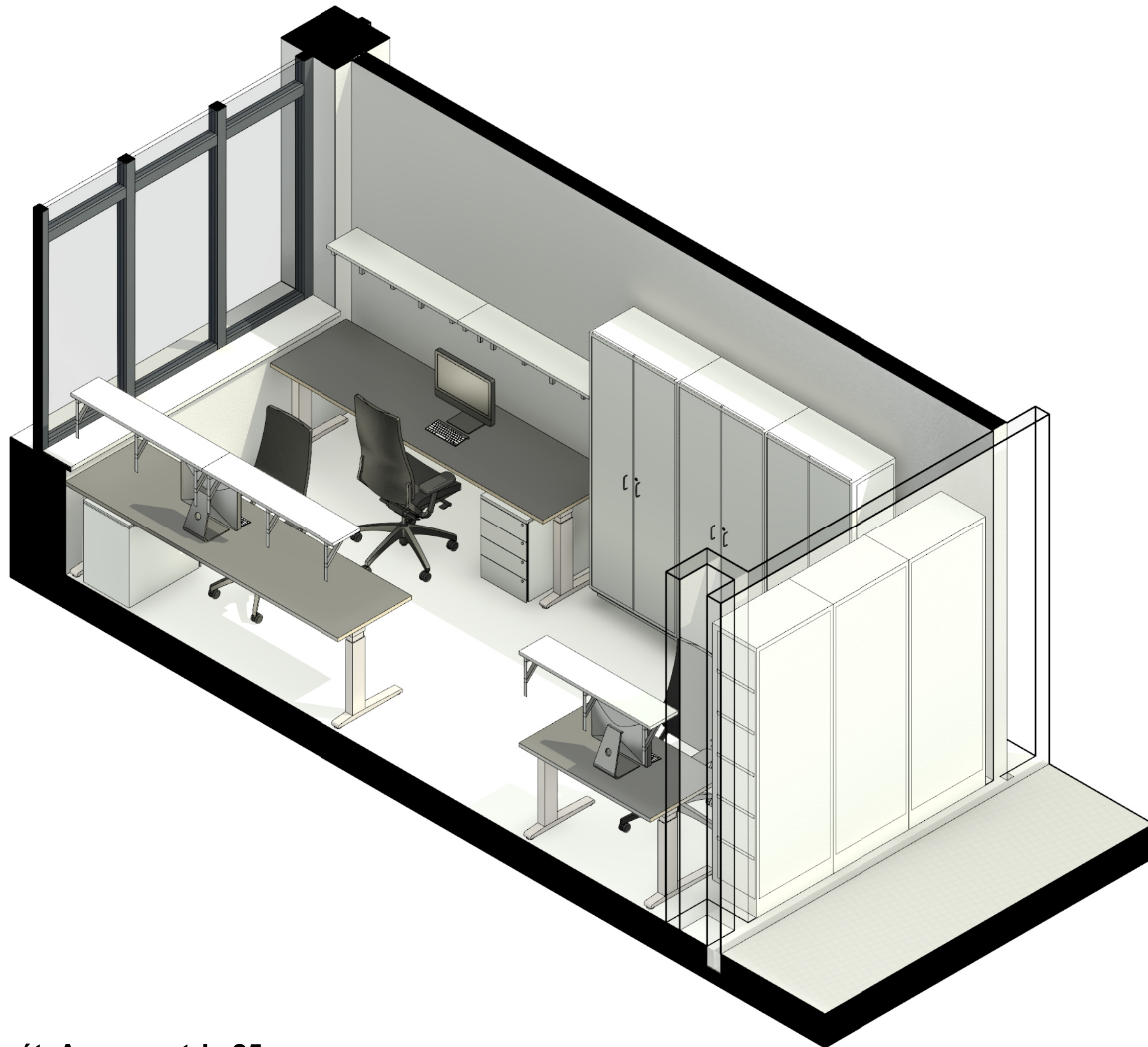
24- UK Rektorát- Axonometria 25a
