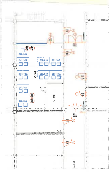
PÓDORYS 2.N.P. - blok B, C M:1:100
