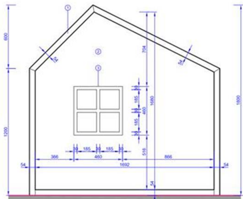
POHLAD ČELNÝ
