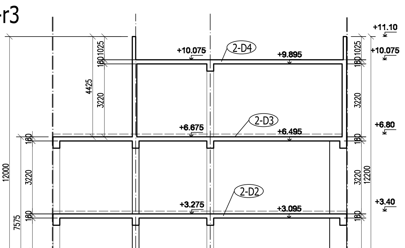
REZ r4-r4 M 1:100
