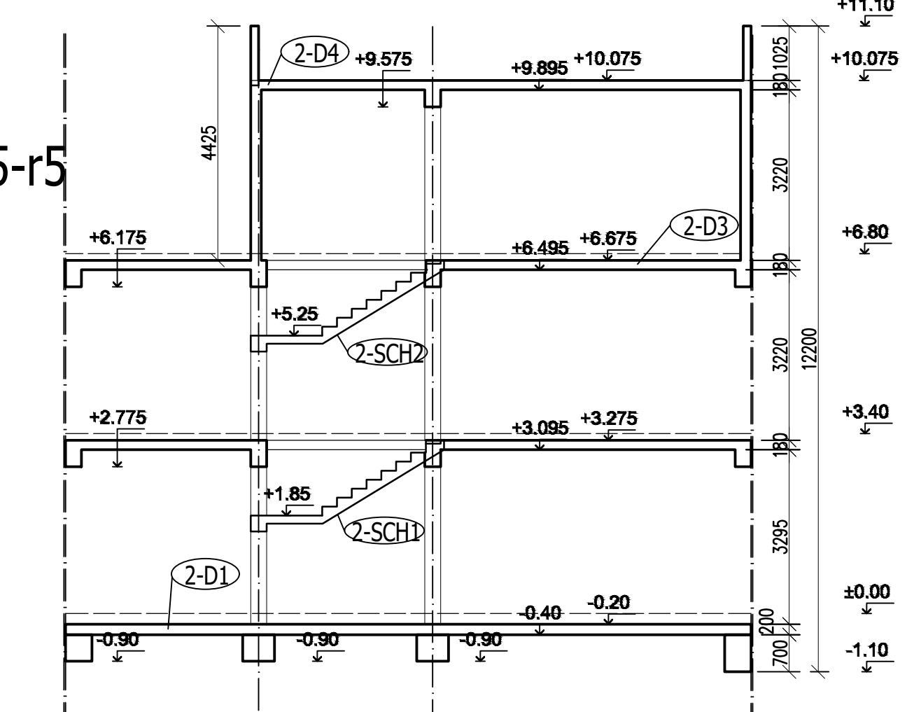
REZ r6-r6 M 1:100
