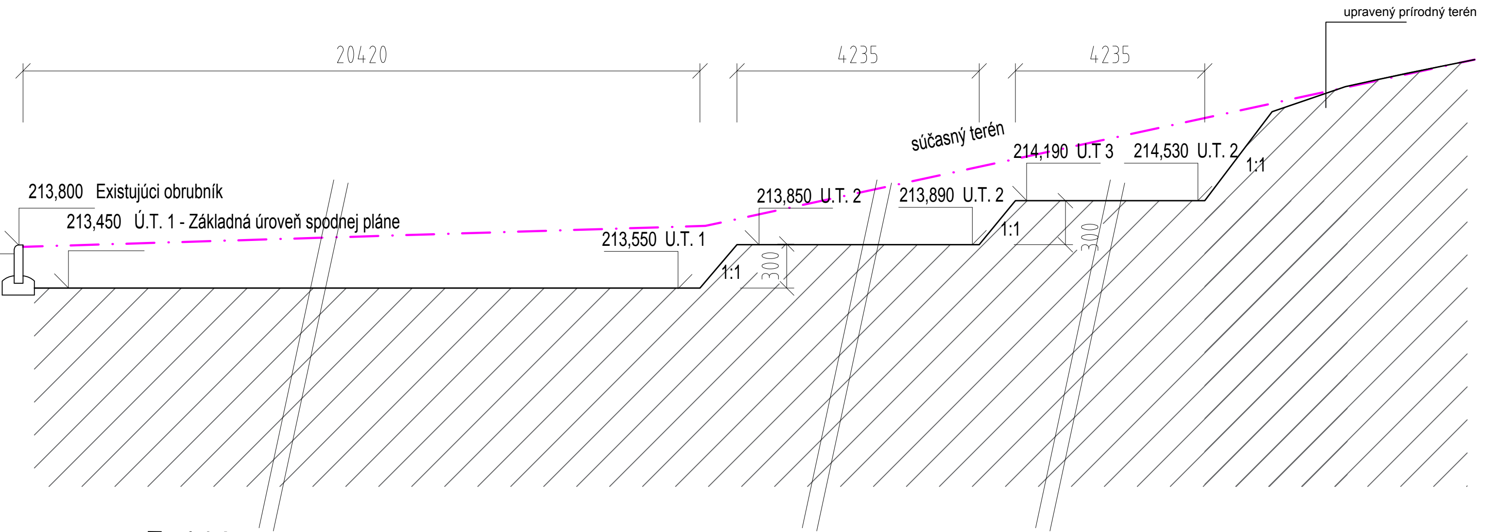
Typický rez A - A' terénnymi úpravami hľadiska
